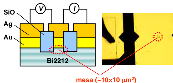
図1 メサ型 IJJ 素子の素子構造(左)と光学顕微鏡写真(右)
