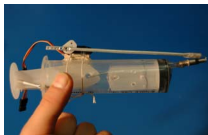
図9 製作した大気採取器
