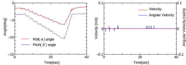
図16 重力補償実験結果
