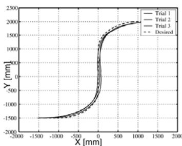
図5 実験結果（人間適応型）
