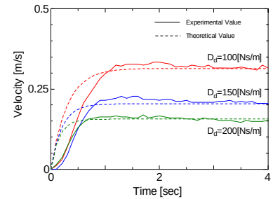
図12 実験結果(理論値との比較)
