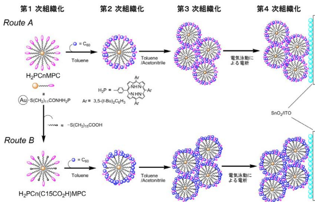
図 3-6 逐次的自己組織化を利用した光電変換系 (「変換と制御」研究成果要旨)
