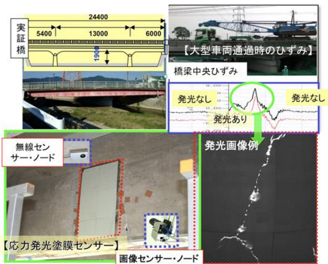
図 3-13 橋梁のモニタリング例
