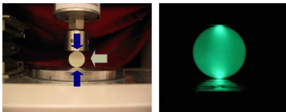
図 3-12 応力発光による応力分布の直接可視化（「変換と制御」研究成果要旨）
