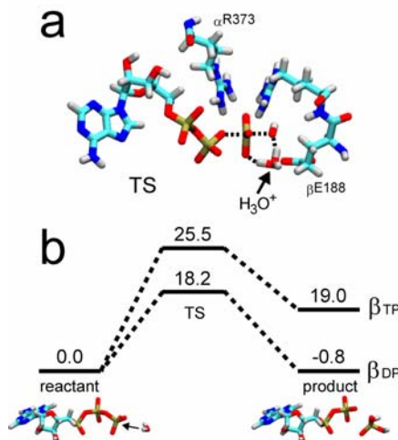
図 4 (a) 反応遷移状態構造と(b) 反応のエネルギープロフィール
