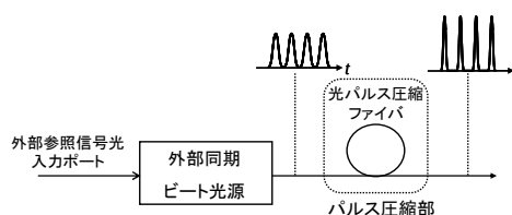
図 1 目指すパルス光源の基本構成。
