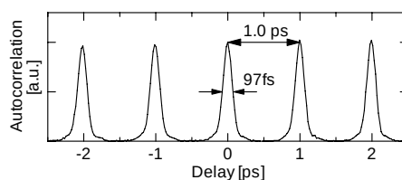
図 4 1 THz 繰り返し光パルス列の自己相関波形。
