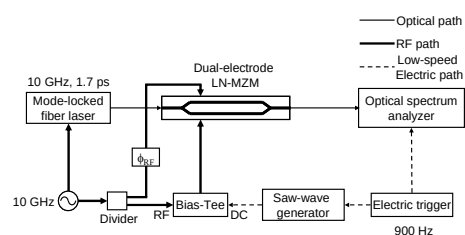
図 11 高感度光パルス特性測定系。
