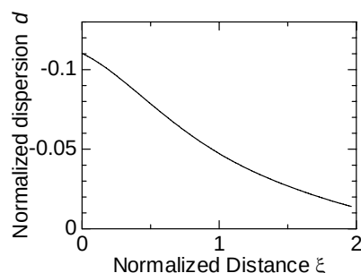
図 2 シミュレーションにより得られた高品質な光パルス列を発生する分散特性
