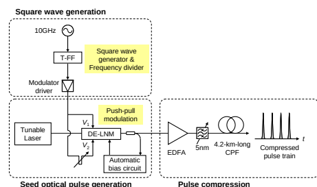
図 10 繰り返し周波数可変・波長可変パルス光源の構成。出力タイミング制
