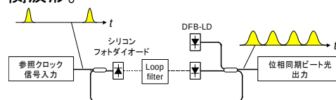
図 5 同期光源の構成概略。DFB-LD: 分布帰還型半導体レーザー。
