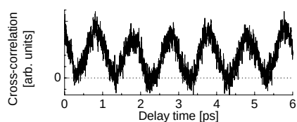
図7 1 THz ビート光と参照信号光の相互相関波形。
