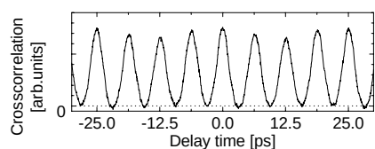
図 9 160 GHz 繰り返し光パルス列と参照信号光の相互相関波形。
