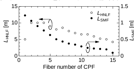
図 3 図 2 の分散特性を模擬するように決定した CPF を構成する各ファイバの長さ。HNLF: highly nonlinear fiber, SMF: single mode fiber.
