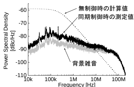
図8 1 THz ビート光の位相雑音スペクトル。
