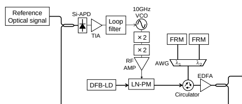
図 12 高スペクトル純度のビート光を出力する低消費電力型同期光源の構成。
