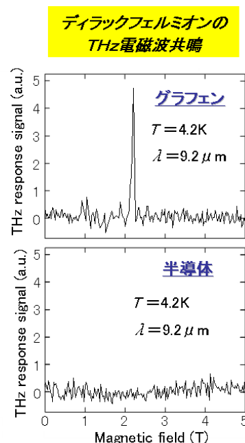
図7. グラフェン(上)と GaAs/AlGaAs(下)の THz 応答信号の磁場依存性。照射THz電磁波の波長は 9.2 \mu m。
