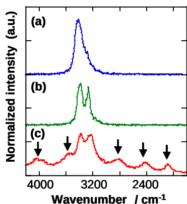
図2 不均一界面への電子増強ラマン散乱の適用。(a)バルク水中、(b)銀表面、(c)銀表面レーザーアブレーション条件。(c)における400cm -1 おきのピークが特徴的(図中矢印)。
