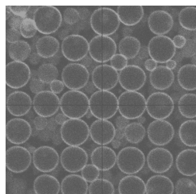
図1：脂質膜のパターニング後にエレクトロフォーメーションを行なった様子。
