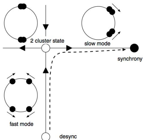
図3: 提案したモデルにおけるクラスタ機構の構造. タイムスケールの違うマニフォールドに沿った運動によって, クラスタ化する.
