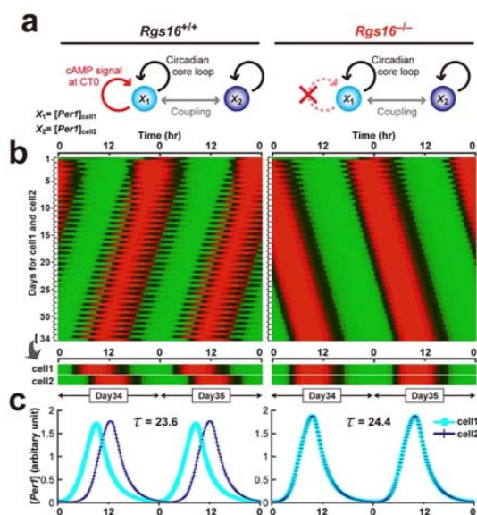
図1: 構築した数理モデルの数値シミュレーション結果. 体内時計を生成する遺伝子制御ネットワークを数理モデル化した. 実験的に観測されてた現象が再現されることを確認した.
