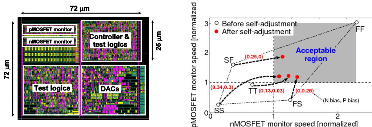
図9: 他のロジックと混載した細粒度特性ばらつき補償回路(左)と、コーナーチップ(SS, SF, FS, TT)の動作速度を補償した結果(右)。
