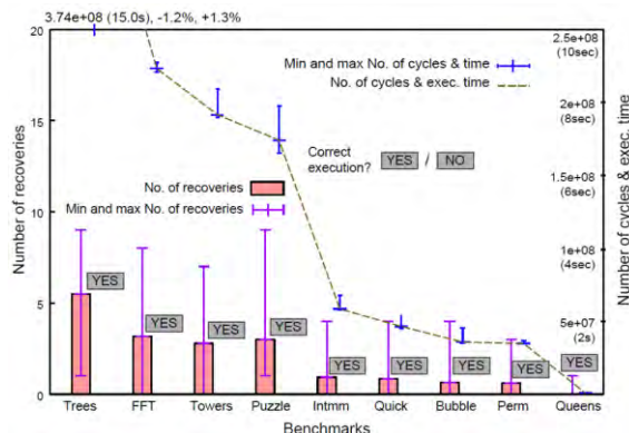
図 6: DARA による適応的多重化実行(左)と試作チップにおける \alpha 線照射評価結果(右)
