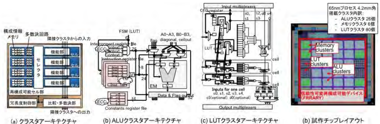
図 5: 信頼性可変再構成可能アーキテクチャ FRRARY ((a)構成要素の基本構成、(b)状態遷移機械による制御が可能な ALU クラスタ、(c)制御処理系やビット演算を実現する LUT クラスタ、(d)試作チップレイアウト)
