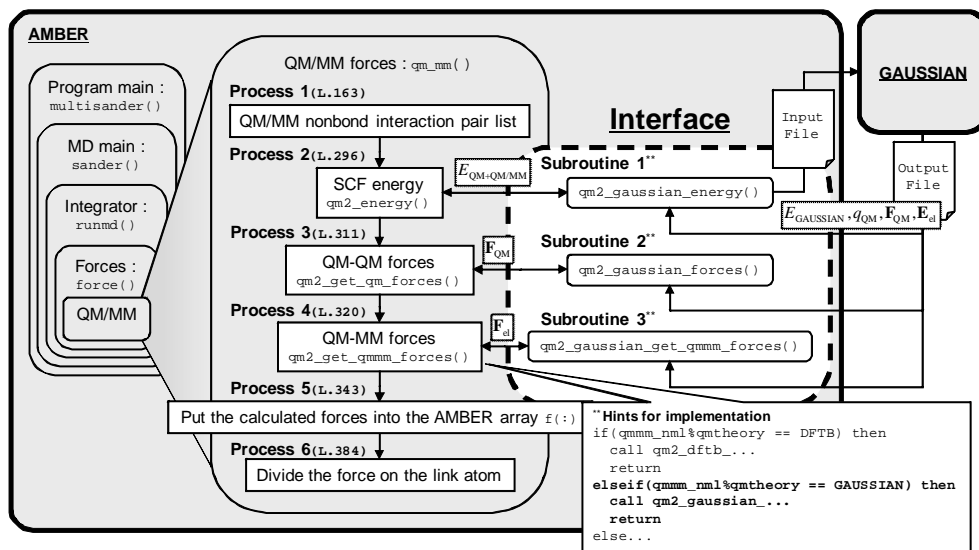
図7 AMBER-GAUSSIAN インターフェイスのアルゴリズム
