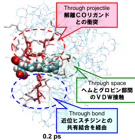
図13 ヘムから周囲残基へのエネルギー緩和経路の分類。励起後 0.2 ピコ秒時点で温度が大きく上昇している残基を強調表示している。励起直後には through projectile と through bond の2経路が主である。nD による 1D 運動反応過程の自由エネルギー
