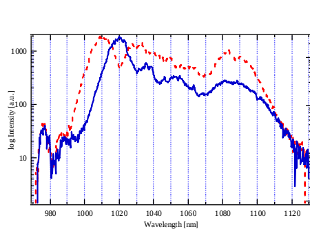
図 16 発振器の出力スペクトル
