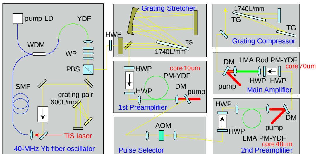
図 20 0.4MHz 50 \mu J ファイバ増幅システムの構成
