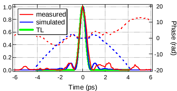
図 22 圧縮後パルスの時間波形(測定と計算)
