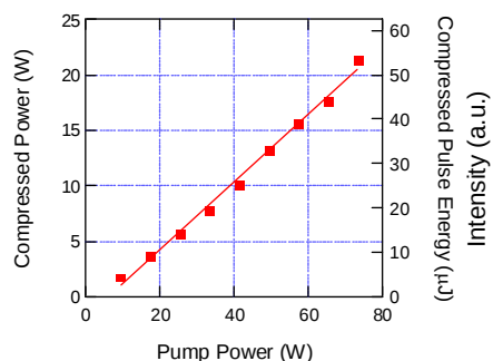
図 21 主増幅器の出力特性
