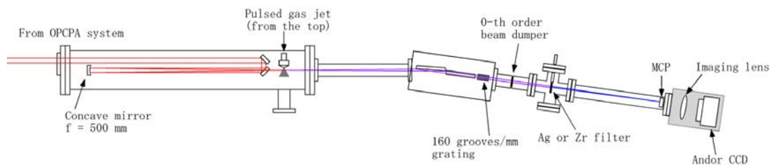
図2. 高次高調波発生系並びに計測系
