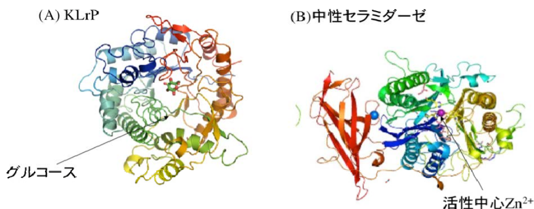
図 2. KLrP は、 \alpha ヘリックスと \beta ストランドを 8 回繰り返す TIM バレル構造を示し、double displacement 機構で水解反応が進行する (Hayashi et al., JBC, 2007; Noguchi et al., BBRC, 2009)。一方、中性セラミダーゼは C 末側のイムノグロブリン様ドメインからなり、Zn イオンを活性中心とする金属酵素である (Inoue et al., JBC, 2009)。
