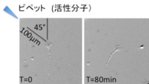
図 4. 神経細胞軸索ガイダンス活性測定法 活性脂質分子をマイクロピペット (内径 1 mm) からパルス状に放出(2~3psi, 2Hz)。理論上、成長円錐の先端に至るガイダンス分子の濃度はマイクロピペット内液の約 1000 分の 1 程度と計算されている。約 10 mm 径の成長円錐は 4~12%の濃度差を感知していると考えられている。この図では、添加したリゾ体ホスファチジルグルコシド(数百 nmol オーダー)を避けるように、成長円錐がリゾ体濃度の低い方向へ移動している (理研・上口研究室との共同研究成果)。
