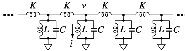
図 15 シュレディンガー方程式の回路モデル
