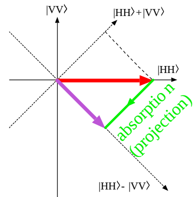
図1 吸収による状態射影
