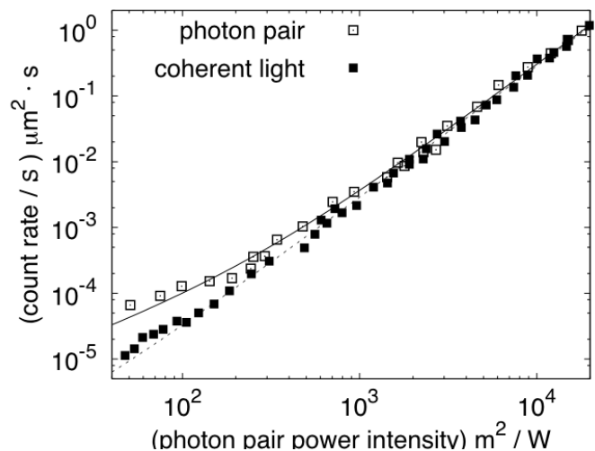
図7 単位時間単位断面積当りのカウント数の光子対光強度依存性(S:入射ビーム断面積)
