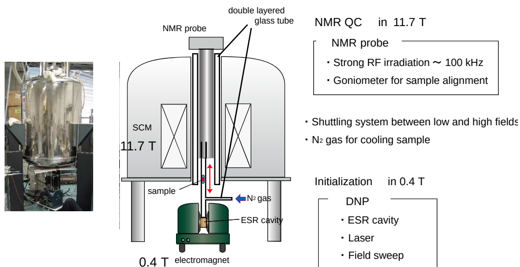
図1-3-1. 光励起三重項低磁場DNP—高磁場NMR フィールドサイクリング装置
