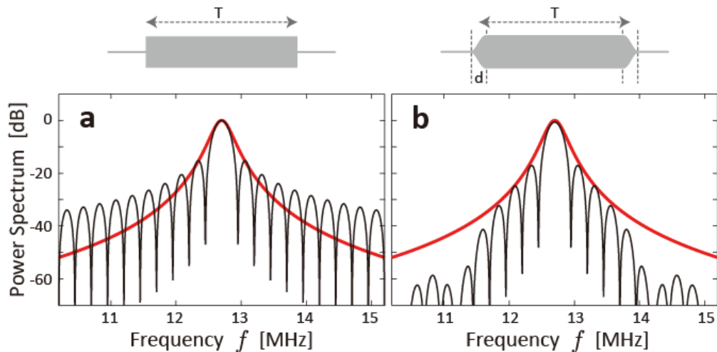
図1-7-2. a 矩形パルスとそのスペクトル, b コサイン立上り・立下りパルスとそのスペクトル
