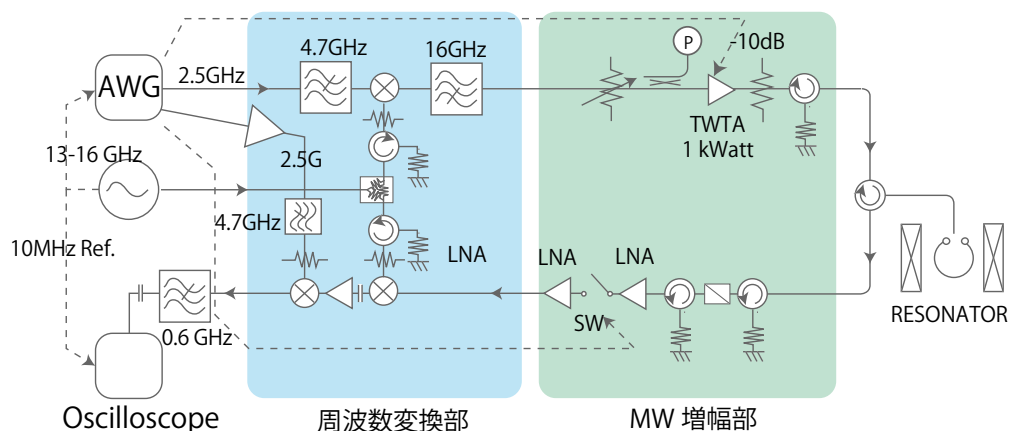
図1-6-1. 任意波形発生器(AWG)ベースのパルス電子スピン多重共鳴装置
