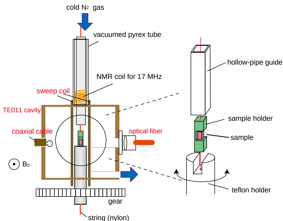
図1-3-2. 光励起三重項DNPによる初期化装置部分
