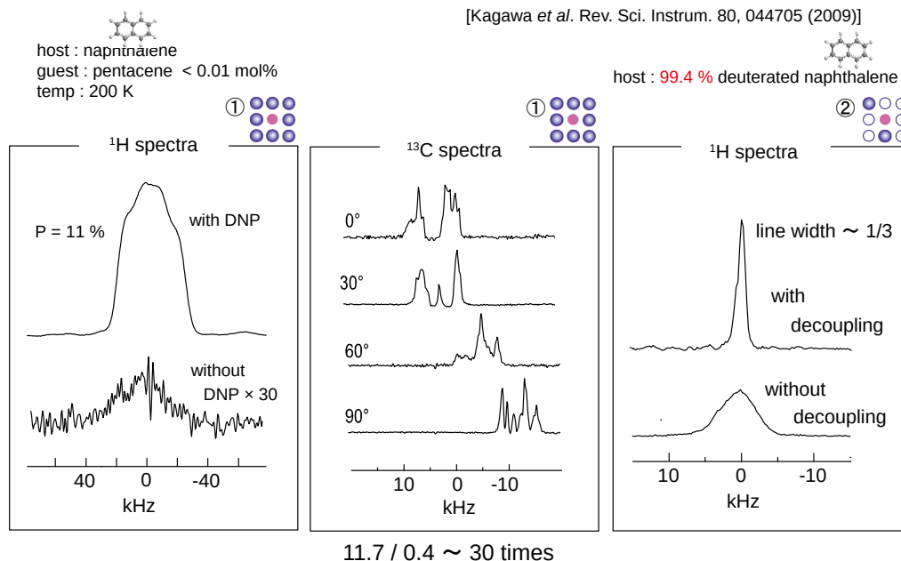
図1-3-4. DNP/NMRフィールドサイクリング装置による高偏極化固体の分光
