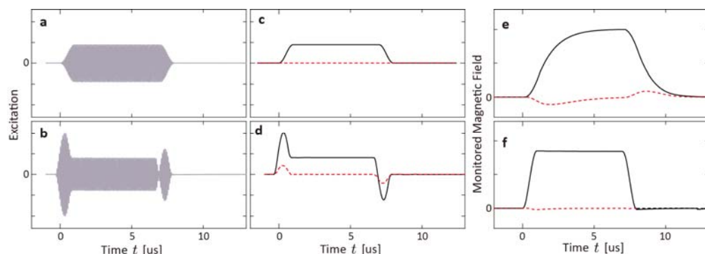
図1-7-4. a コサイン立上り・立下りパルス、b 補償パルス、c d はab のIQ 振幅、ef はaを補償せずに印加した場合と補償してbを印加した場合の共振器内磁場のIQ 振幅の実測値
