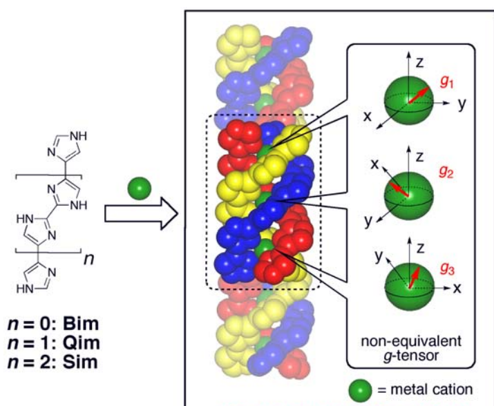
三重螺旋対称性を利用して、電子スピンをもつ金属イオンの周りの対称性を制御する、g-tensor engineering アプローチ
