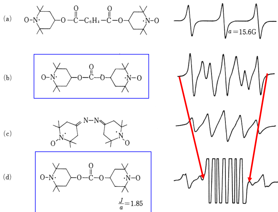
図 2-1-1. 等方的電子スピン交換相互作用の大きさと溶液中の超微細構造スペクトルに現れる biradical の交換相互作用由来の分裂。
