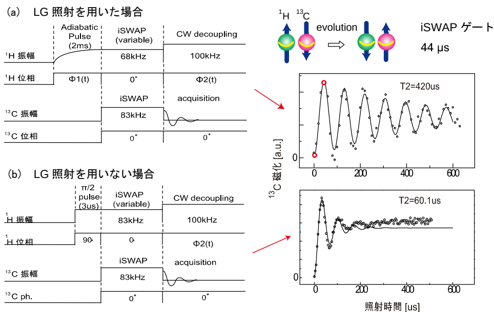
図1-2-2. LG照射による2量子ビット iSWAP ゲート(L-アラニン)
