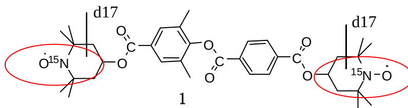
図 2-2-5. genuine g-engineering で分子設計し、新規に合成した 2-electron qubit 系分子の分子構造。
