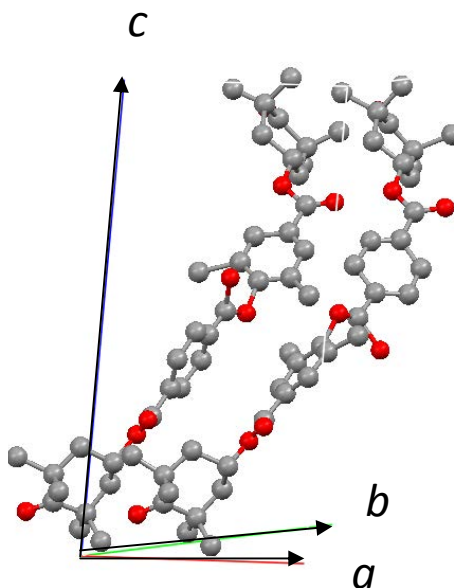
図 2-2-7. genuine g-tensor engineering で分子設計した 2-electron qubit 系分子 (1) 2 分子の結晶格子内での配向を結晶軸 a , b , c , との関係で模式的に示す。
