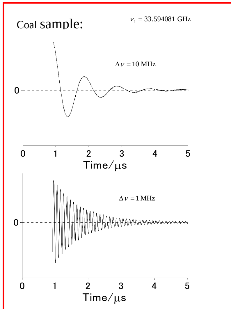
図 2-2-3. 周波数の異なる電子スピンの相対位相が制御されている様子示す、スピネコーの減衰曲線。抱絡線は、coal sample の減衰曲線に対応する。
