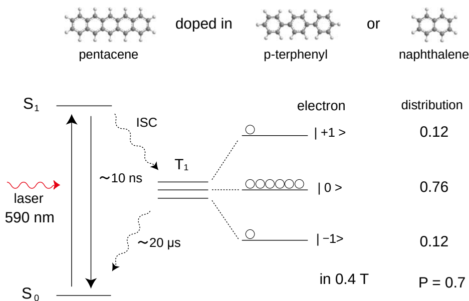
図1-1-1. ペンタセンのエネルギー準位
