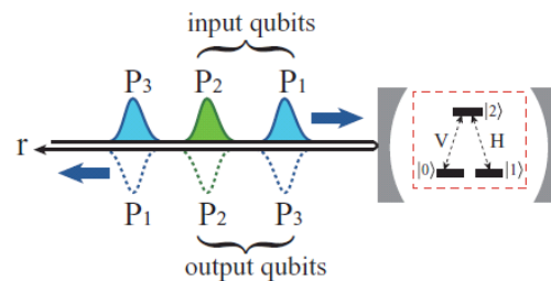
図4-4. 決定論的光子-光子エンタングルゲート。
