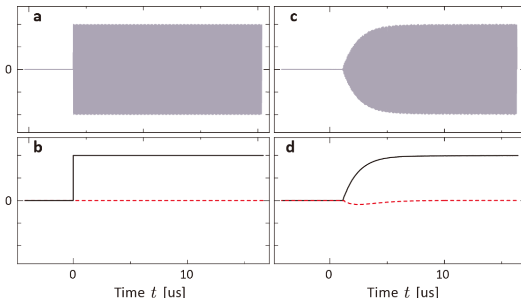
図1-7-3. a 伝達関数測定用ステップ正弦波入力、c 応答、bd はac のIQ 振幅
