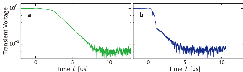
図1-7-6. 共振器パルス補償によるデッドタイム短縮
