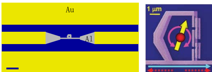
図4-1. マイクロ波伝送線路と結合した磁束量子ビット。右は磁束量子ビット部分の拡大図。
