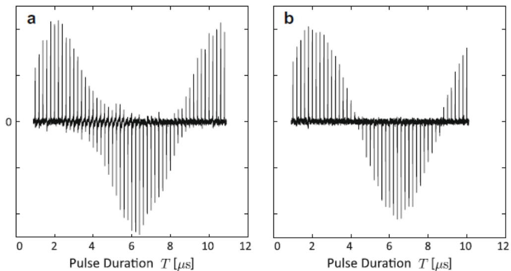
図1-7-5. ラビ振動に現れる位相ランジェント(a 共振器補償無し、b 共振器補償あり)
