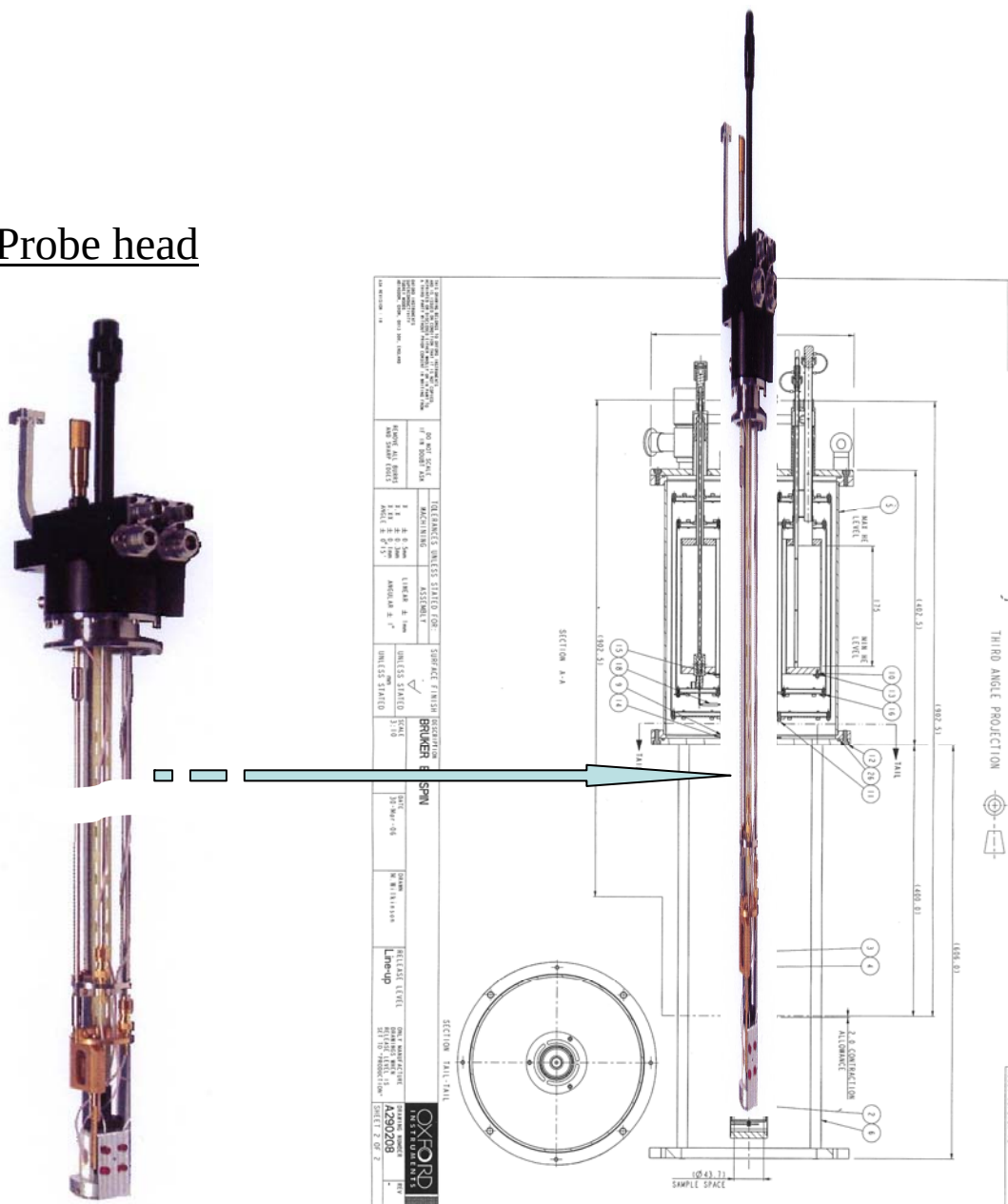
図 2-2-1. coherent dual 電子スピン-電子スピン二重共鳴(CD-ELDOR)用 probe head の概観及び第 1 号クリオスタットの内部を示す。
