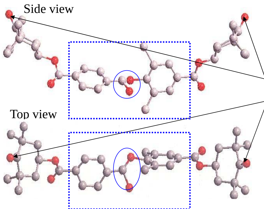
図 2-2-6. 対応する two-electron spin-qubit を望む濃度でホスト格子内に取り込む、第 3 世代のホストジケトン(1a: 図 2-1-3 参照)。交換相互作用は、極めて小さく、電子スピン磁気双極子相互作用の 100 分の 1 程度である。結晶構造の対称性、及び分子スピン分子構造上、ホスト格子中には、磁氣的に区別できる分子スピンは、1 種類存在する(下図 2-2-7)。
