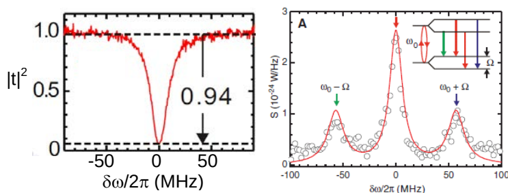
図4-2. 共鳴蛍光。(左) 共鳴周波数における透過光の抑制。(右) 非弾性散乱スペクトルにおいて観測された Mollow 三重項。
