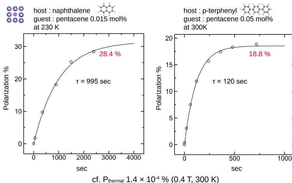
図1-1-2. 左ナフタレン結晶ホスト、右 p-テルフェニル結晶ホスト
