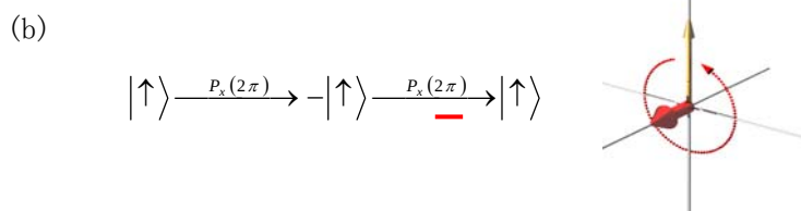
図 2-2-4. 電子スピン qubit のスピノールを直接観測した、ラジオ波・マイクロ波パルス系列(top)と電子スピンのブロッホ球の二つの極を回るときに 4\pi 周期性を示す(b)、電子スピンエコー信号((a)下)。
