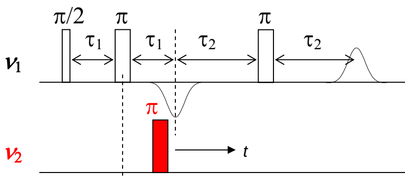
図 2-2-8. 分子スピン系 1 の電子スピン間磁気双極子相互作用テンソルを実験的に決めた、4-パルス ELDOR のパルス系列。
