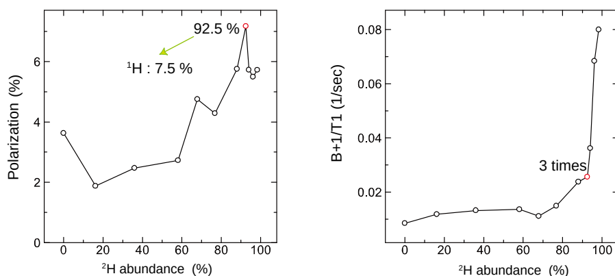
図1-1-3. 到達偏極率(左)とビルドアップレート(右)の重水素化率依存性
