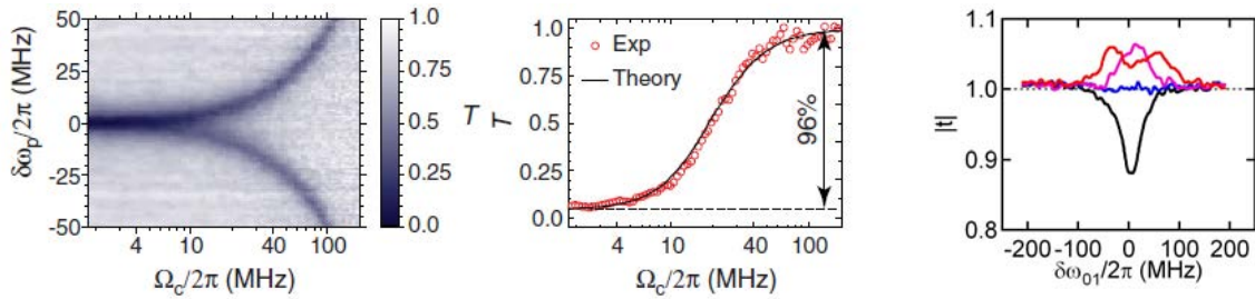
図4-3. 人工3準位系を用いた実験。(左) Autler-Townes 二重項の分裂。(中) 共鳴周波数におけるプローブ光透過強度のポンプ強度依存性。(右) ポンプ光により生成された反転分布の引き起こす誘導放出によるプローブ光の増幅。透過係数が1より大きくなりゲインが得られている。
