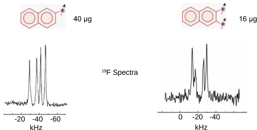
図 1-4-2. フッ素核スピン量子ビットの初期化後のNMRスペクトル
