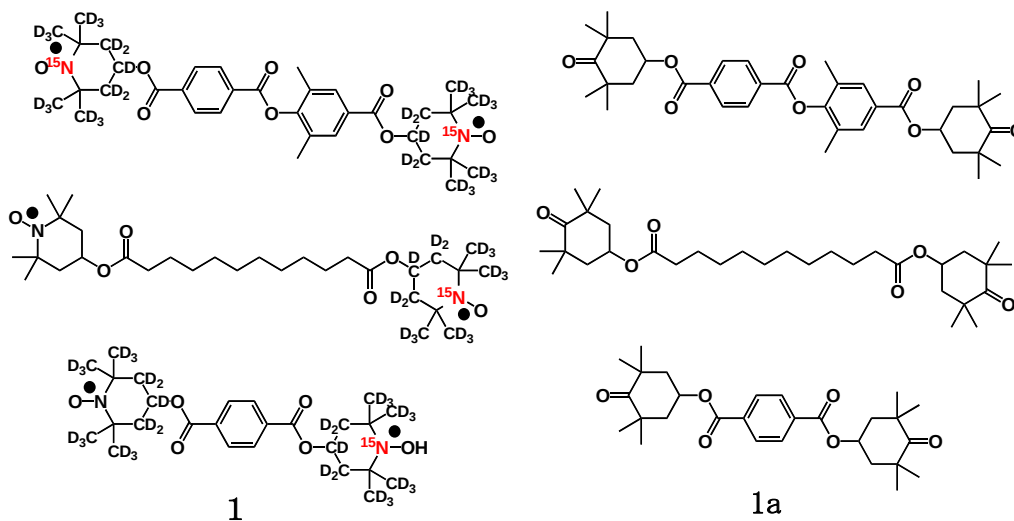
図 2-1-3. 代表的な 2qubit 分子スピン(biradicals:左)と対をなす反磁性分子ジケトン(右)。
