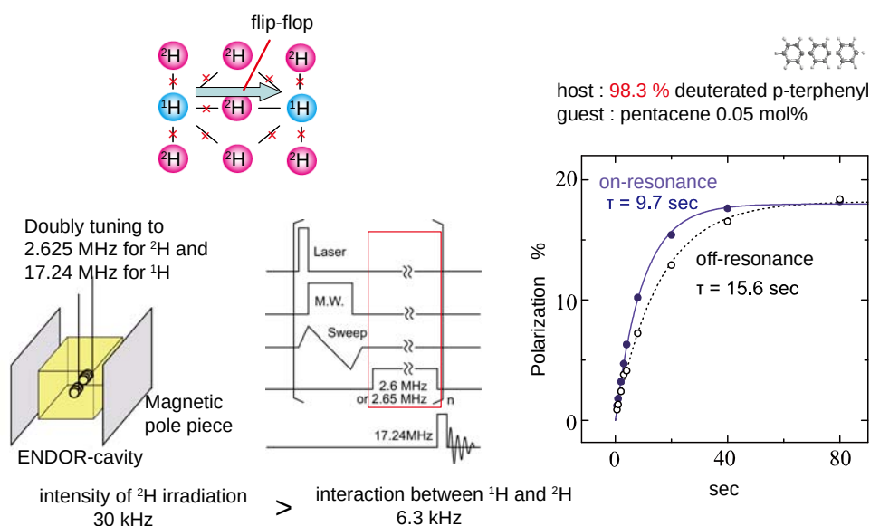
図1-1-4. 重水素デカップリングによるプロトン間スピン拡散の高速化
