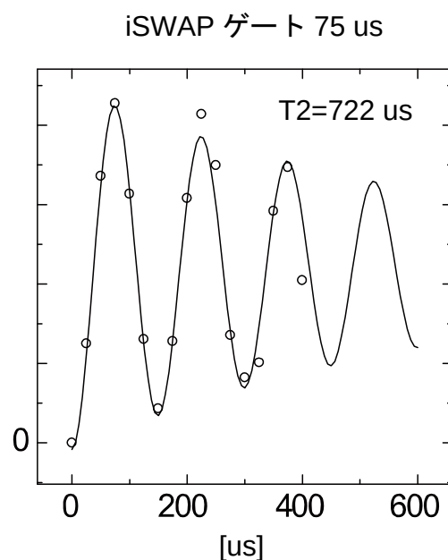
図 1-4-1. 初期化可能な 2 量子ビット分子とそれを用いた LG 照射による iSWAP
