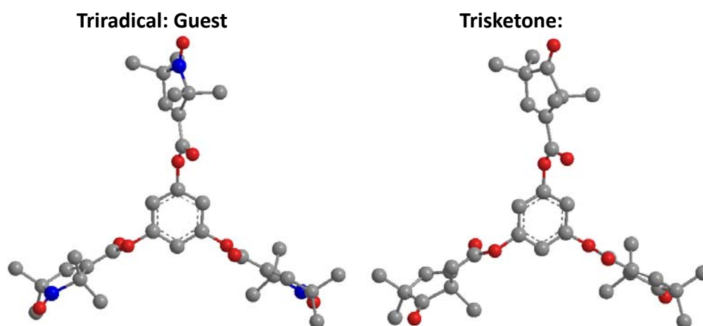
図 2-1-4. 3-qubit 弱交換相互作用分子系 Triradical (左)、及びトリスケトンホスト分子 (右) の分子構造 (X 線構造解析の結果にもとづく)。窒素核は、すべて ^{14}\text{N} 核である。ここでは、電子磁気共鳴スペクトルの単純化のためのスピンサイト NO の ^{15}\text{N} 同位体置換はされていない。Triradical (左) において、青色球は ^{14}\text{N} 核を示す。
