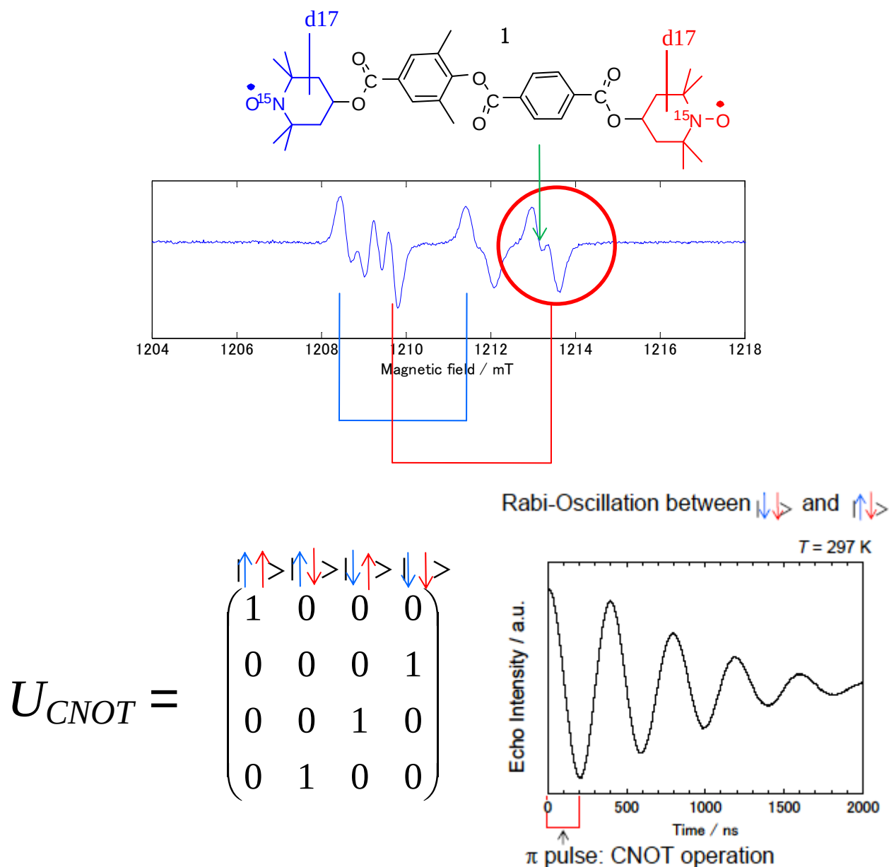
図 2-2-9. 分子スピンの電子スピン 2-qubit 系で観測された最初の CNOT ゲートをしめす Rabi 振動(下図、右)。
