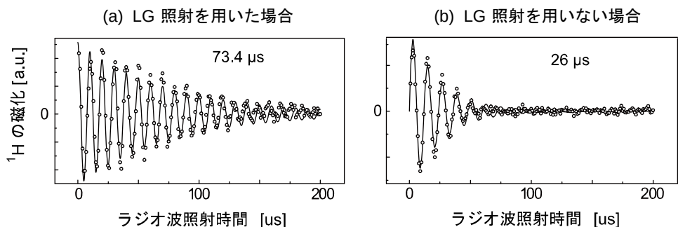
図1-2-1. LG 照射による1量子ビット回転ゲート(L-アラニン)
