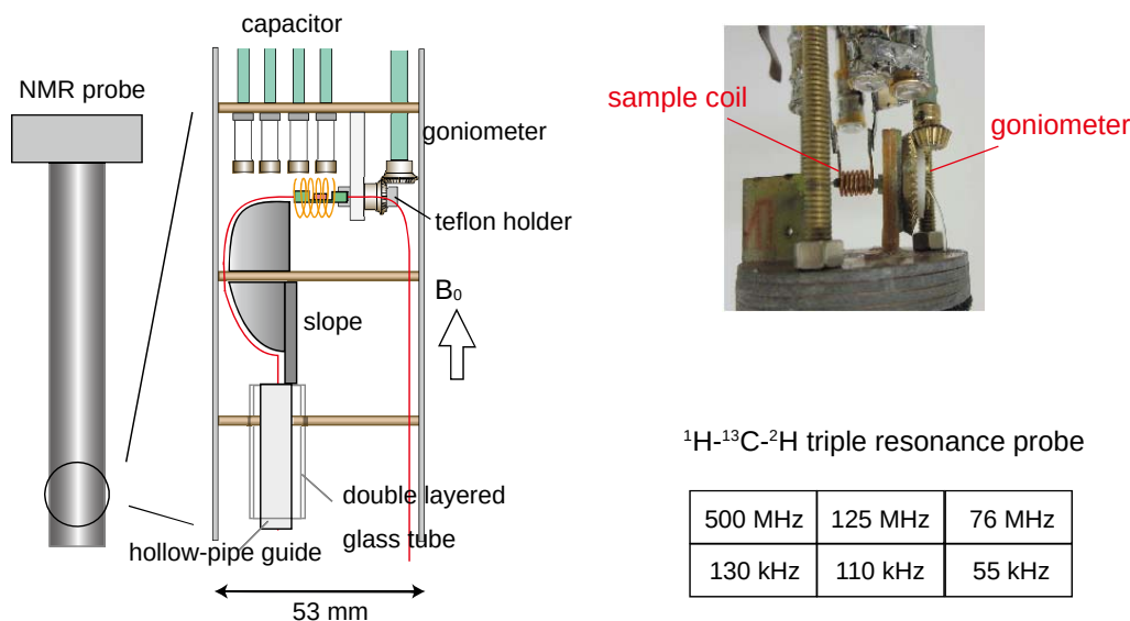
図1-3-3. 高磁場NMRプローブ部分
