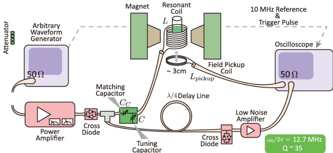
図1-7-1. パルス補償の実験配置
