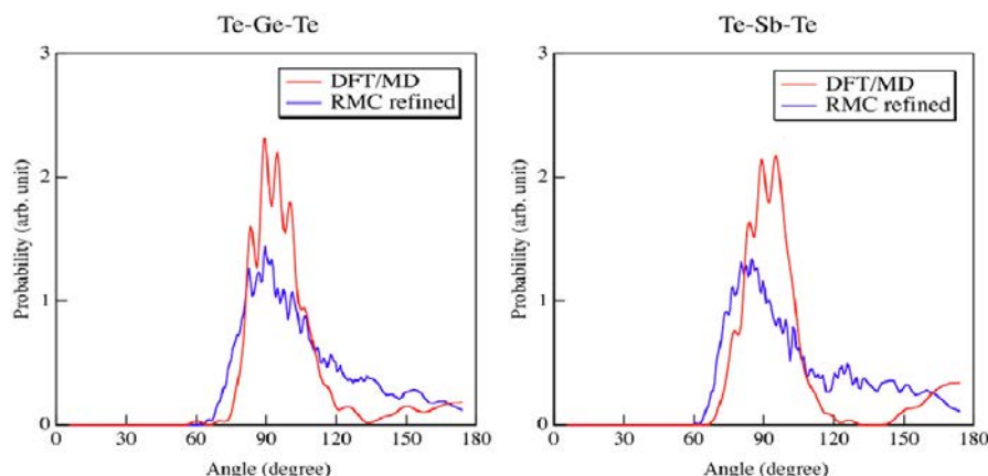
図 26 DFT/MD 計算および RMC モデリングによる構造リファイン後の \text{Ge}_2\text{Sb}_2\text{Te}_5 アモルファスの角度分布。
