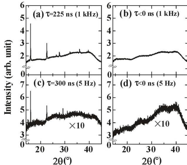
図 13 遅延時間 \tau が、(a) \tau = 225 ns と (b) \tau < 0 ns の X 線回折パターンのスナップショット。比較のため、マイクロビームを使用せず、5 Hz の繰り返しでのデータ取得した以前の測定結果を (c) と (d) に示す。
