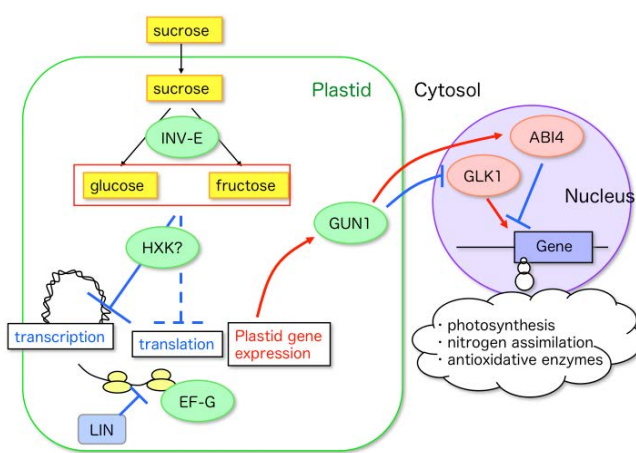
図 10 インベルターゼを介したプラスチド遺伝子発現調節機構。葉緑体内での糖代謝が、光合成関連、窒素代謝関連の遺伝子発現を制御する機構（予想図）。葉緑体内のインベルターゼ（INV-E）が、ショ糖をグルコースとフルクトース（ヘキソース）に分解する。これまでヘキソキナーゼ（HXK）が糖（ヘキソース）センサーとして機能していることが示されており、葉緑体局在の HXK も同様の機能をもつ可能性がある。HXK により、葉緑体ゲノムにコードされた光合成関連遺伝子の転写および翻訳を抑制される。それらがさらに GUN1, GLK1, ABI4 などのタンパク質を介した葉緑体から核への逆行性シグナルによって、核ゲノムにコードされた光合成および窒素代謝関連の遺伝子発現を制御する。
