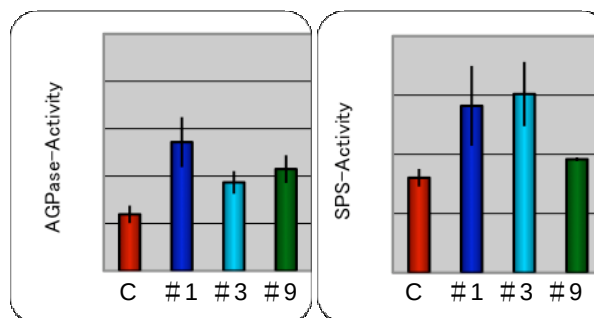
図 4 Dof1 形質転換バレイショ。コントロール植物（C）と Dof1 形質転換体（#1、#3、#9）の塊茎における ADP グルコースピロホスホラーゼとショ糖リン酸合成酵素と活性。
