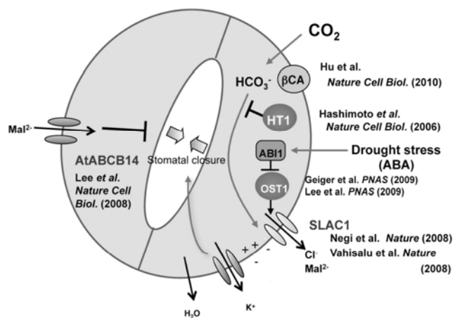
図 16 これまでに同定されている孔辺細胞における \text{CO}_2 シグナル伝達因子と関連因子。
