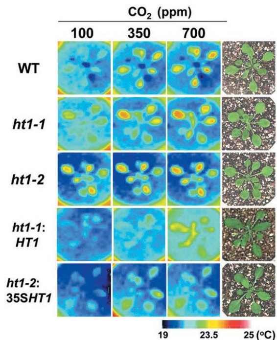
図 15 ht1 株の CO 2 応答。さまざまな CO 2 濃度における葉表面温度を観察した。2つの ht1 変異株 ( ht1-1 と ht1-2 ) とともに低 CO 2 環境で高い葉表面温度を示す。この表現型は野生型の HT1 遺伝子を発現させることで見られなり ( ht1-1 : HT1 )、CaMV35S プロモーターを用いて野生型の HT1 を過剰発現させた場合には、逆に、高 CO 2 環境で低い葉表面温度を示した ( ht1-2:35SHT1 )。
