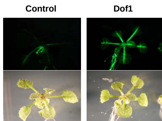
図 2 Dof1 形質転換植物の代謝バランスの可視化。APR1 プロモーター制御下の GFP 遺伝子を野生型シロイヌナズナと Dof1 形質転換シロイヌナズナに導入し、アンモニウムを含む培地を用いて強光下で生育させ、GFP 遺伝子の発現を比較した。
