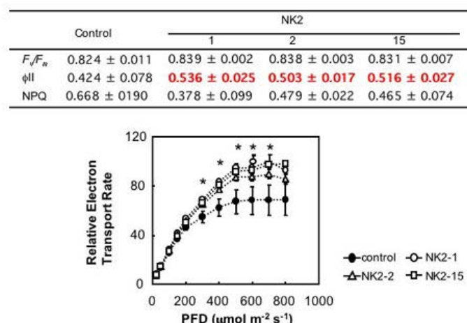
図13 NADK2高発現イネ系統（NK2）における光合成電子伝達系の亢進。光化学反応の最大量子収率 F_v/F_m については、NADK2高 発現植物とコントロール植物との間に差異は見いだされなかったが、光化学系IIにおける有効量子収率（化学エネルギー生産に使用された光エネルギーの比率）や光合成電子伝達速度については、高光強度条件下のNADK2高発現イネで高い数値を示した。また、光化学系IIで発生した余剰な電子を熱として放出する。熱放散（NPQ）の値が、NADK2高発現植物では低い数値を示した。これらの結果は、NADK2高発現イネでは、電子を受け取るNADPプールが増大する事により光合成電子伝達系が促進され、熱として放出される余剰エネルギーが減少していることを示している。
