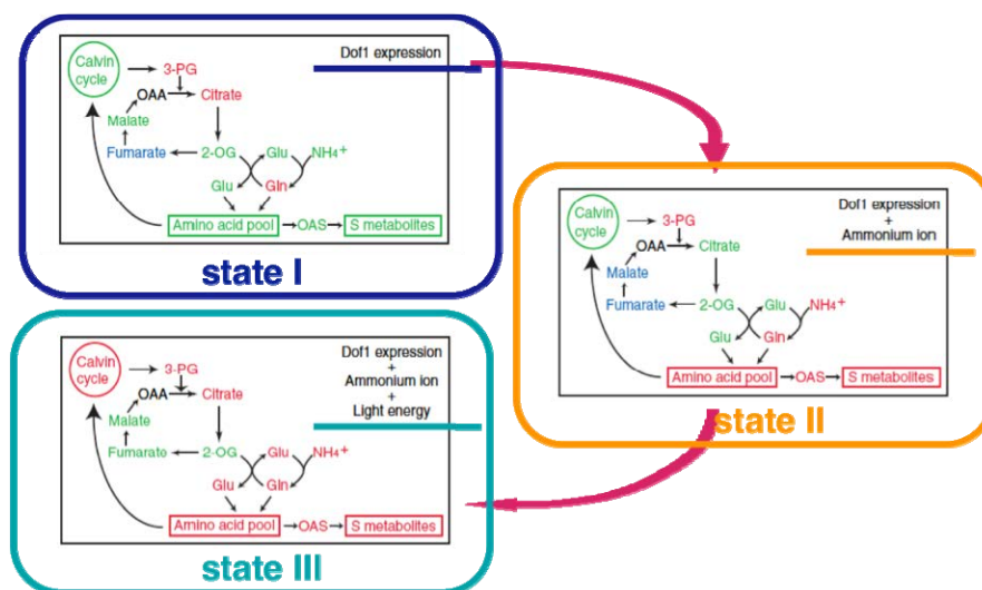
図1 Dof1 シロイヌナズナで見られる無機イオン同化経路の同調的強化のモデル図。Dof1 植物体では、最初に窒素同化に必須な炭素代謝物のレベルの上昇が引き起こされている (state I)。この時、アンモニウムイオンが供給されると窒素の同化が促進され遊離アミノ酸のレベルの上昇を引き起こす。遊離アミノ酸のレベルの上昇に伴い硫黄同化も活性化している (state II)。窒素代謝物と硫黄代謝物の含量の増加は光合成による炭酸固定の促進を促す。Dof1 シロイヌナズナにおいて窒素代謝物と硫黄代謝物の含量の増加が見られる生育条件下で、光の強さを強くすると炭酸固定量に有意な違いが見られる (state III)。野生型株に比べて、含量の多い代謝物や活性化された代謝路が赤で示されている。
