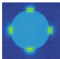
図 3-4-2 4 個のスロットを 持つ円筒内外の 磁界
