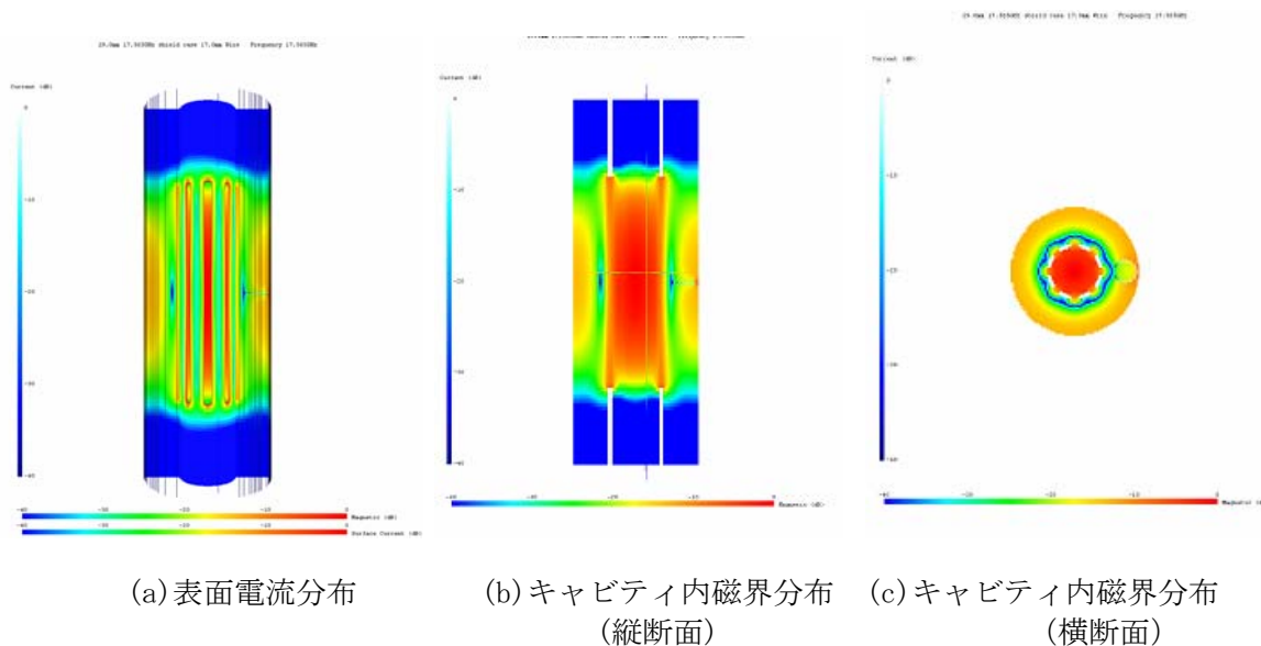
図 3-4-7 Ku バンド円筒シールド付 SAR の磁界分布
