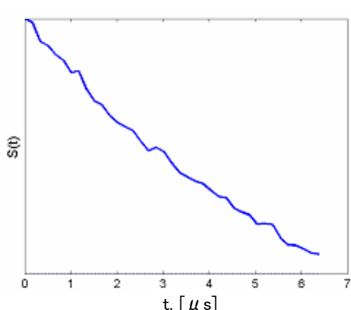
図 3-4-9 円筒シールド付き SAR 使用による \gamma 線照射石英砂内の E^{\wedge} センター
