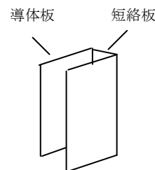
図 3-4-3 蓋としての 終端短絡平行平板 回路(フィン)
