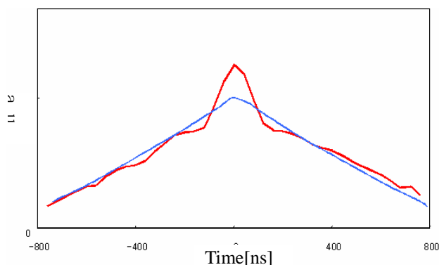
図 3-4-5 \gamma 線照射石英砂の E' センター — 本研究による測定値 周波数 : 9.2GHz 温度 : 60K パルス列 : 6 パルス \pi/2 パルス : 25ns — Peter P. Borbat らによる測定値[3]
