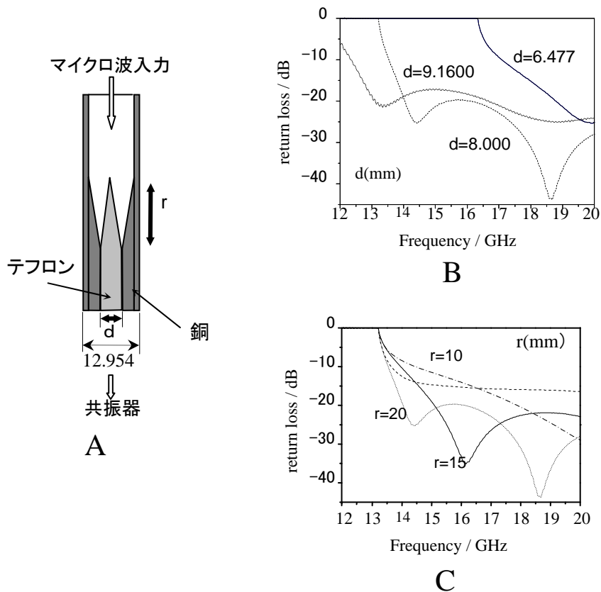
図3-2-6 Gordon Coupler (A)、と数値解析によるReturn Lossの絞り幅 d およびテーパ長さ r 依存性 (B, C)
