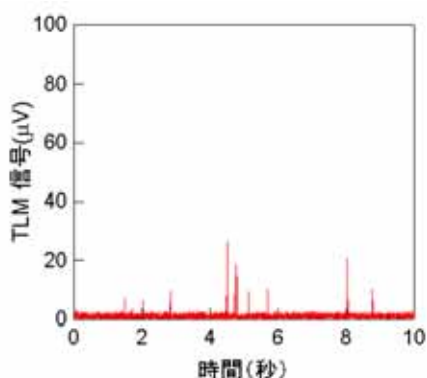
図 26 ナノチャンネル中のカウンティング
