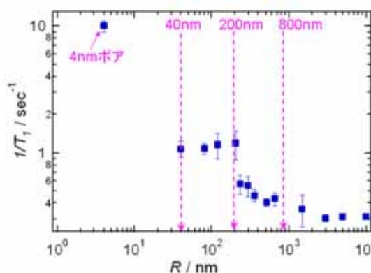
図 13 ^1\text{H} - 1/T_1 値の空間サイズ依存
