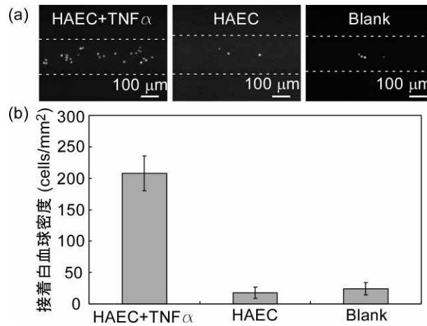
図 10 血管内皮細胞を培養したマイクロチャンネル内での白血球接着実験結果。(a) 蛍光画像。(b) 白血球密度の比較。
