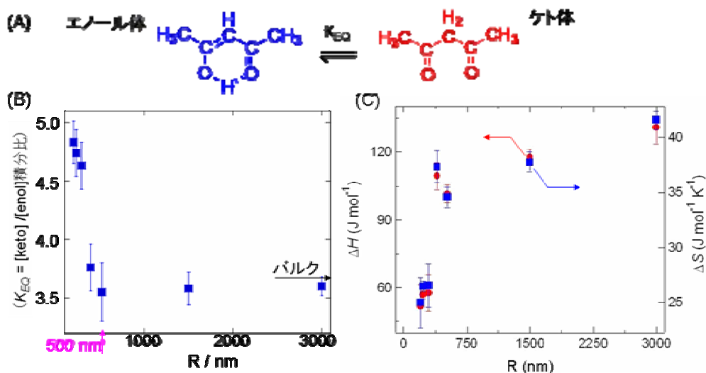
図 20 (A) keto-enol 互変異性化反応 (B) K_{\text{EQ}} の空間サイズ依存 (C) \Delta H , \Delta S の空間サイズ依存
