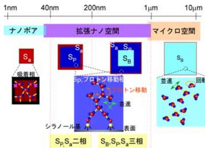
図 16 水分子挙動と三相モデル
