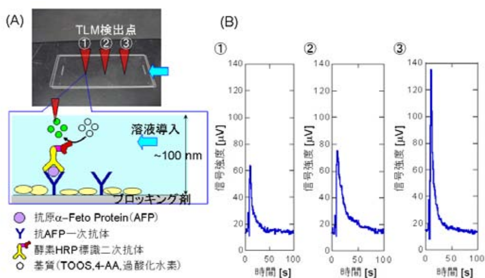
図 30 (A) ナノイムノアッセイ用チップと反応系 (B) 各位置における TLM 信号強度
