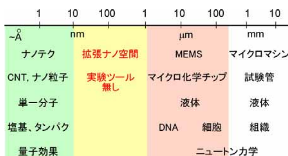
図1 サイズ階層と拡張ナノ空間
