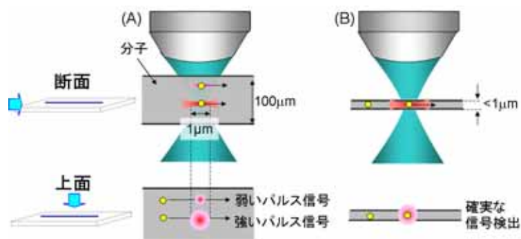
図 25 (A)マイクロチャンネル, (B)ナノチャンネル内分子カウンティングにおけるパルス信号強度変化
