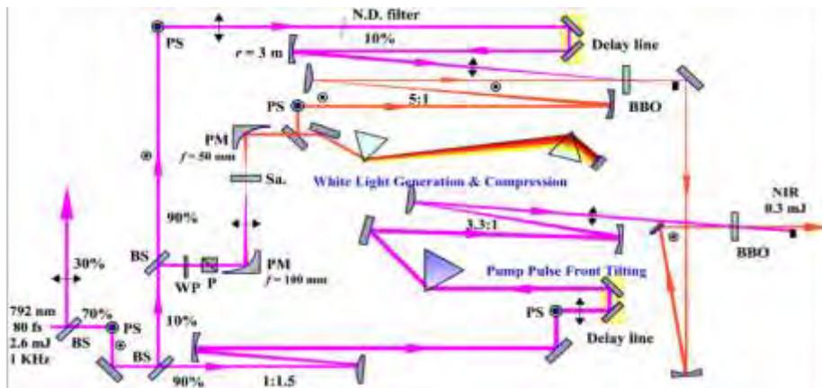
図4 製作された近赤外光パラメトリック増幅器の光学レイアウト図
