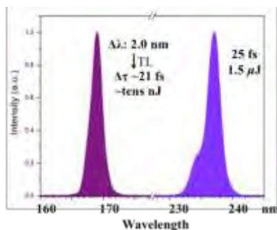
図5 NIR-OPAと2倍波から発生した深紫外光と真空紫外光のスペクトル
