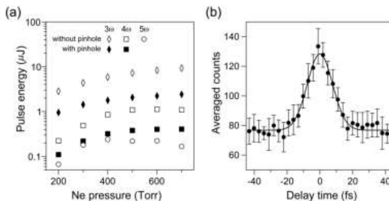
図 9 (a) 3\omega (ひし型), 4\omega (四角), および 5\omega (白丸)のパルスエネルギーの圧力依存性。白色のシンボルは、ピンホール未使用時、対して黒色のシンボルはピンホール使用時のパルスエネルギーを示す。(b)キセノンの非共鳴二光子イオン化により得られた 4\omega と 5\omega の相互相関関数。黒丸は実測値、実線は半値全幅 18 fs のガウス関数を示す。
