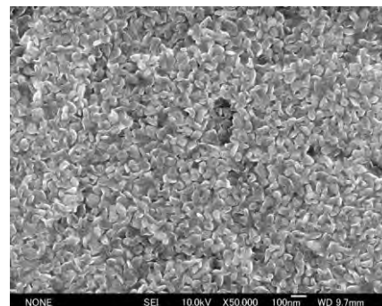
図 21 TiOPc (10nm) + TiOPc (100°C, 10nm)の SEM 画像
