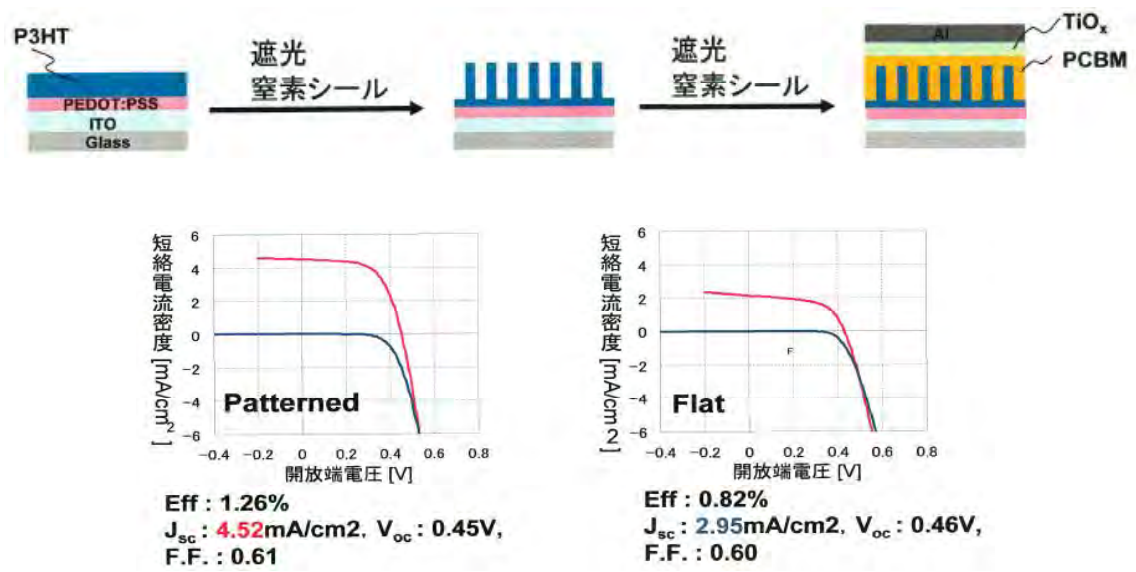
図 22 ナノインプリント構造 (Patterned) セルと平面ヘテロ構造 (Flat) セルの電流-電圧特性
