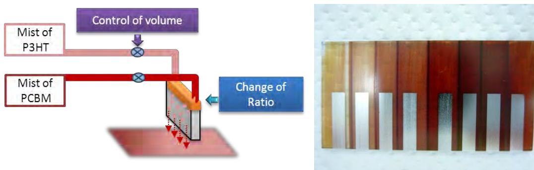
図 18 二重噴霧装置(左)とP3HT/PCBM 傾斜薄膜 (右)
