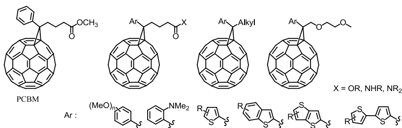
図 1 新規に合成した各種 PCBM 誘導体
