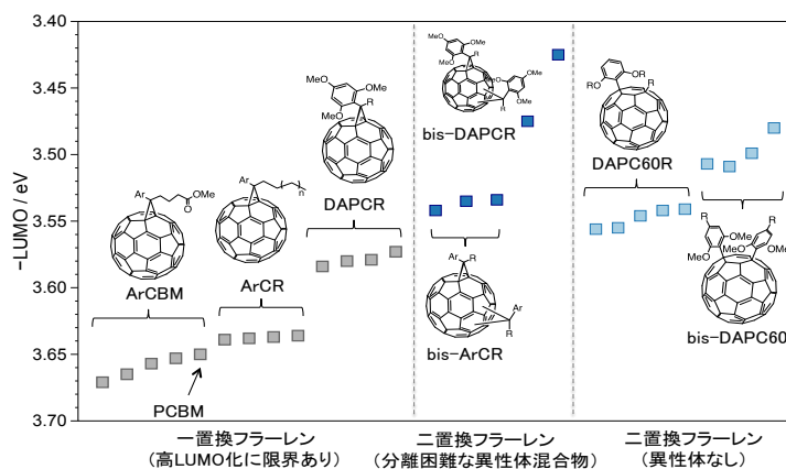
図 2 開発したフラーレン誘導体の LUMO エネルギーレベル
