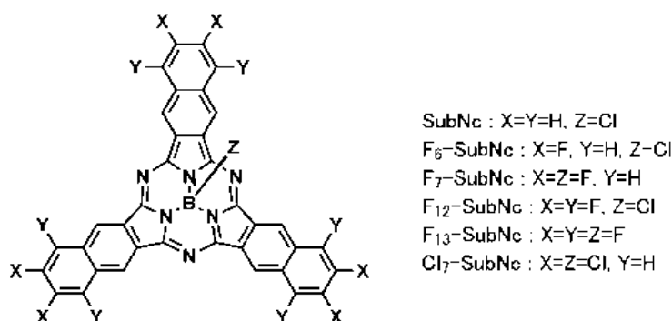
図 10 合成したハロゲン化 SubNc 誘導体
