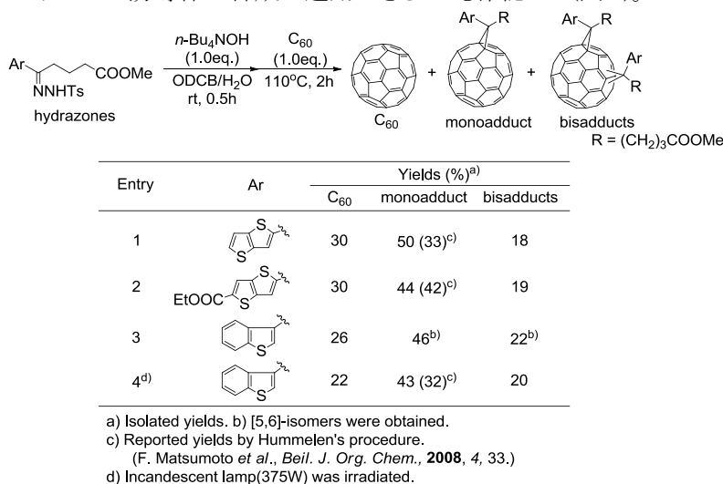
図 5 水系二層系反応を用いたメタノフラーレン誘導体の新規合成法
