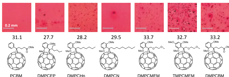
図 3 フラーレン誘導体の表面自由エネルギー(mJ/m²)と薄膜モルフォロジー
