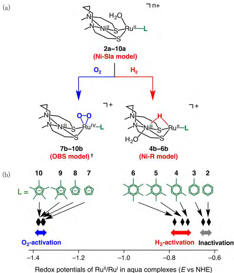
図16 ニッケルルテニウム錯体による水素と酸素の活性化、†: a model complex for \text{O}_2 -bound species
