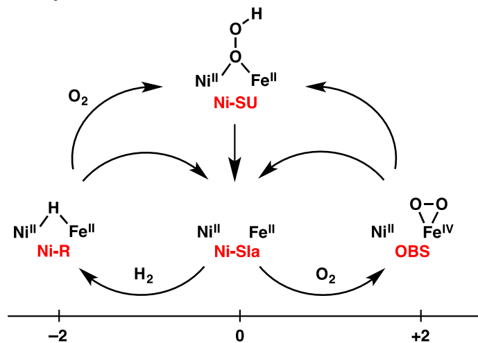
図1 酸素耐性[NiFe]ヒドロゲナーゼの H 2 と O 2 に対する反応性、横軸の目盛りは、Ni-Sla を基準[0]としたときの、NiFe 中心に電子が入った個数を表している。電子は負の電荷をもつため、電子が入るほうがマイナスの目盛り、電子が出るほうがプラスの目盛りとなる。Ni-R:EPR-silent reduced state、Ni-Sla:EPR-silent active state、OBS:O 2 -bound species
