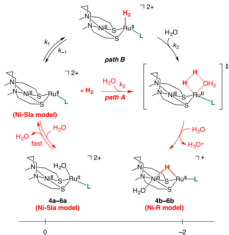
図19 水素活性化反応のメカニズム
