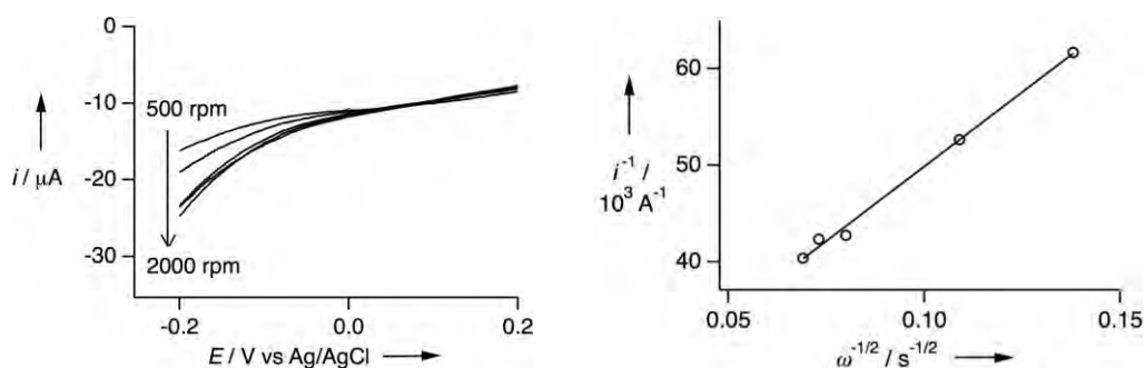
図 28 (a) \text{Ni}^{\text{II}}\text{Ru}^{\text{IV}} ペルオキシ錯体 10b による酸素還元反応の回転リング-ディスク電極を用いた電気化学的測定、(b) Koutecky-Levich プロット
