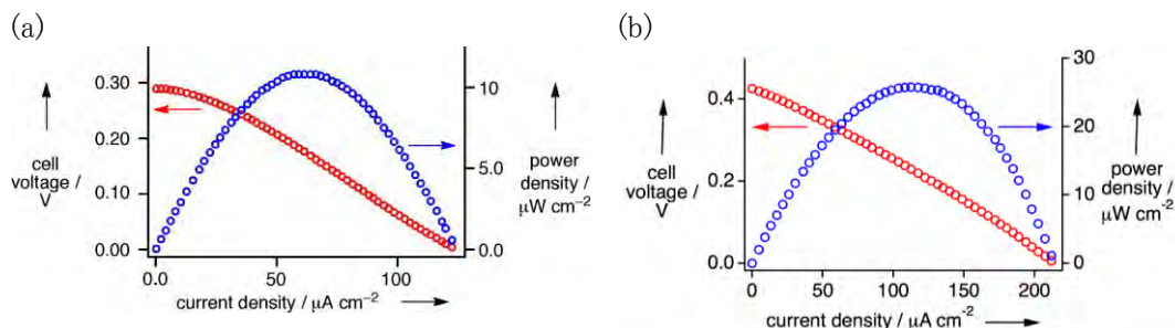
図25 (a) 分子燃料電池の電流-電圧曲線と電流-電力曲線(アノード: \text{Ni}^{\text{II}}\text{Ru}^{\text{II}} ヒドリド錯体 6b 、カソード: \text{Ni}^{\text{II}}\text{Ru}^{\text{II}} ヒドリド錯体 6b )、(b) 分子燃料電池の電流-電圧曲線と電流-電力曲線(アノード: \text{Ni}^{\text{II}}\text{Ru}^{\text{II}} ヒドリド錯体 6b 、カソード: \text{Ni}^{\text{II}}\text{Ru}^{\text{IV}} ペルオキシ錯体 10b )
