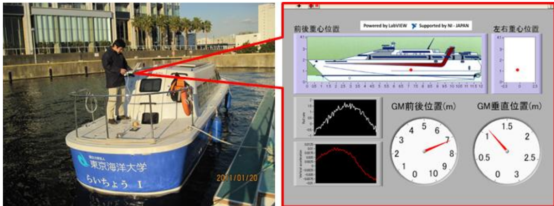
船舶用三次元重心検知システム(転覆防止技術)
