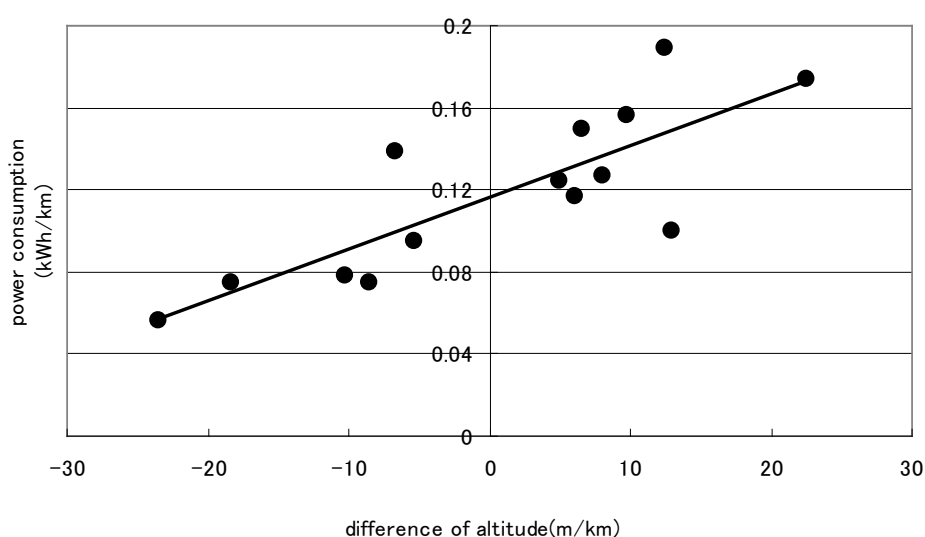
図 3-3-7-6 電気自動車の実測走行データ
