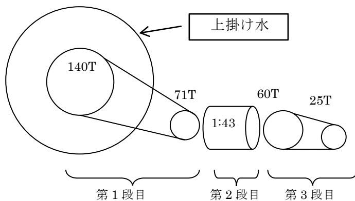
図 3-3-1-10 増速機構の構成略図。T は歯数を表す。
