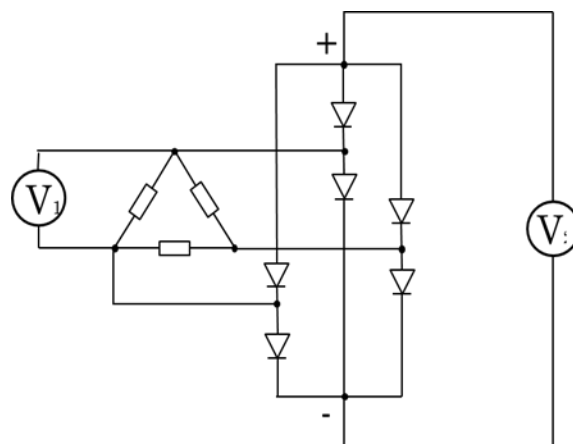
図 3-3-5-6 解放電圧測定回路図
