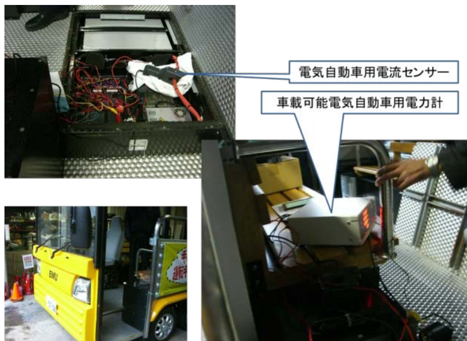
図 3-3-7-5 使用した電気自動車および電力消費量測定状況
