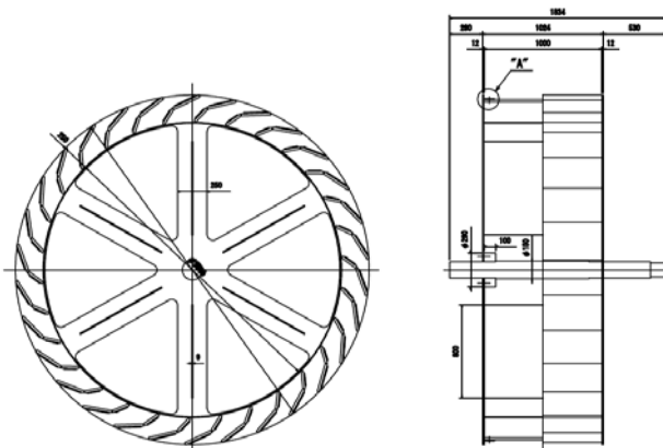
図 3-3-2-3 上掛け水車の側面図（左）と正面図（右）
