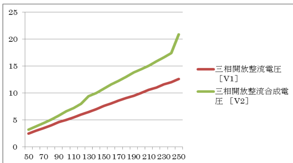
図 3-3-5-7 回転を変化させた場合の出力の変化
