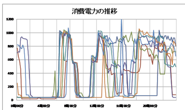
図 3-3-6-3 家屋における消費電力の時間経過
