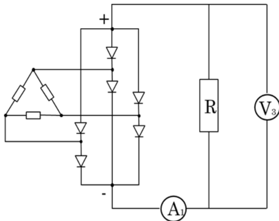
図 3-3-5-9 抵抗器 R を入れた場合の電流・電圧測定の回路図
