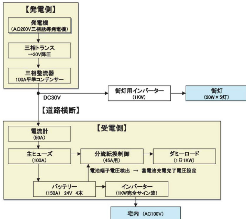
図 3-3-2-2 螺旋水車で用いた電力制御回路
