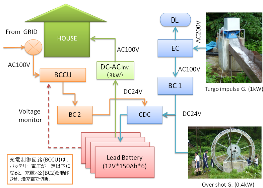
図 3-3-6-2 需給バランス調整のために開発した回路のブロックダイアグラム。EC:電力制御盤、BC1,2: バッテリー充電器 1,2、CDC: 充放電コントローラ、DC-AC Inv.: DC-AC インバータ、BCCU: 充電器制御ユニット、DL: ダミーロード。BCCU はバッテリー電圧が一定以下になると充電器 2 を動作させ、系統電力 (GRID) を用いてバッテリーを充電する。
