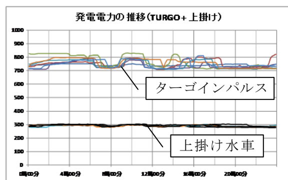
図 3-3-6-4 2 台の水車発電機の出力の時間経過
