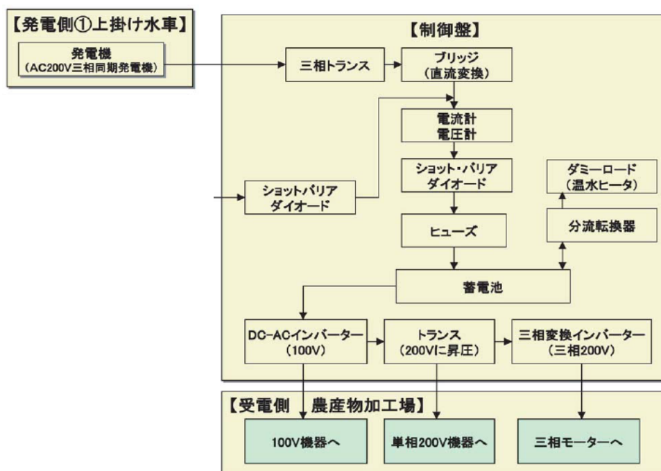
図 3-3-2-5 上掛け水車で用いた電力制御回路
