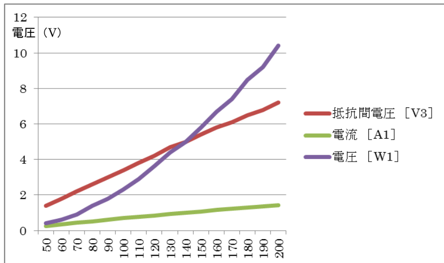
図 3-3-5-10 回転を変化させた場合の出力の変化
