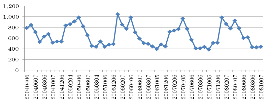
図 3-3-1-2 対象農家における月間電力消費量の推移 (2004年6月～2008年10月)
