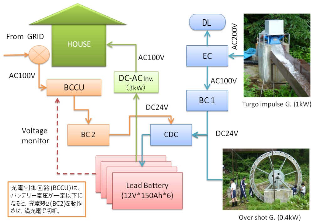
図 2-3-5 電力自給システムにおける需給バランス調整回路
