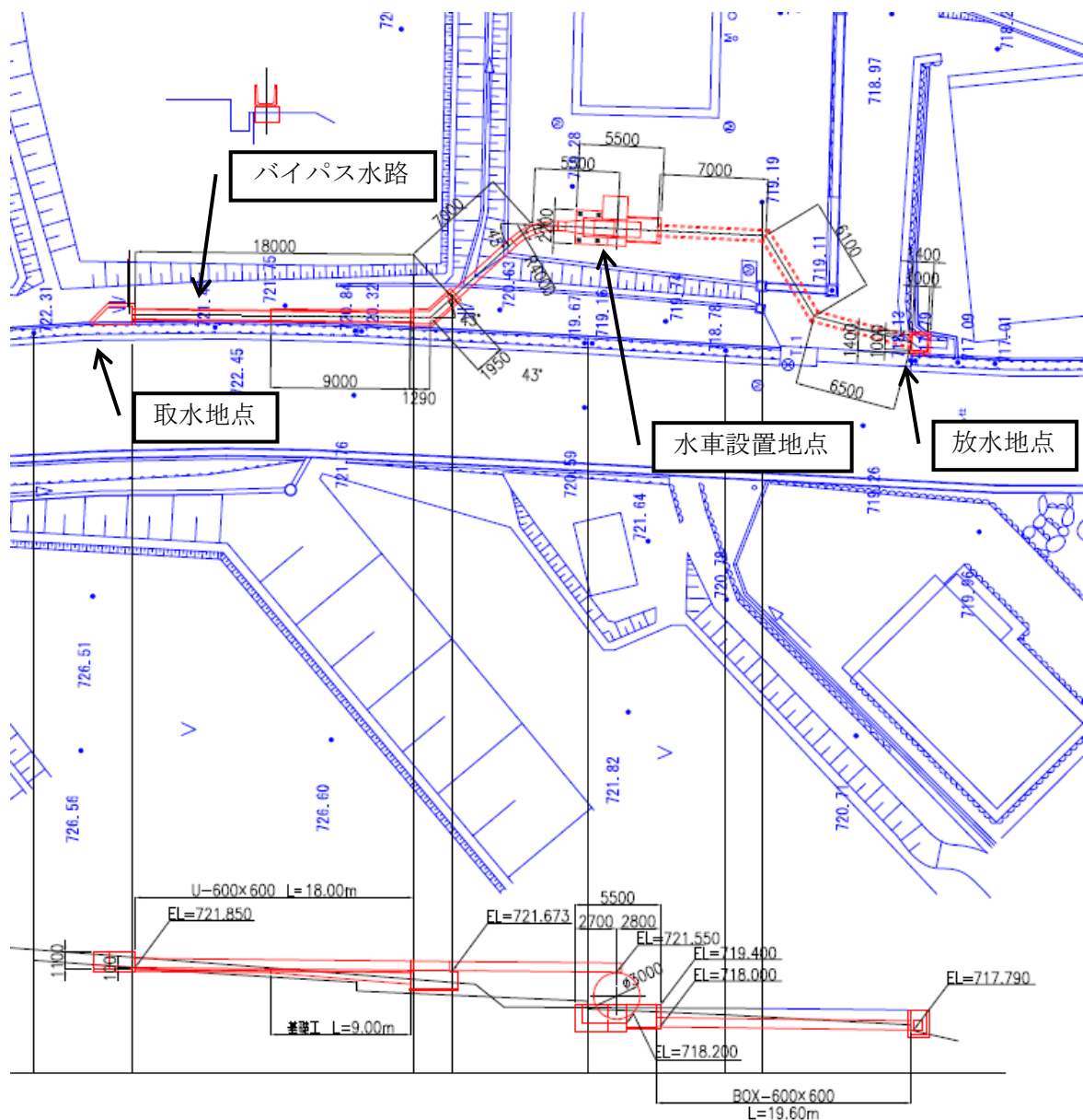
図 3-3-2-4 上掛け水車設置の施工図。上段が平面図、下段が縦断図。
