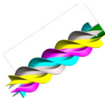
図 3-3-12-7 4 枚羽根完成イメージ)
