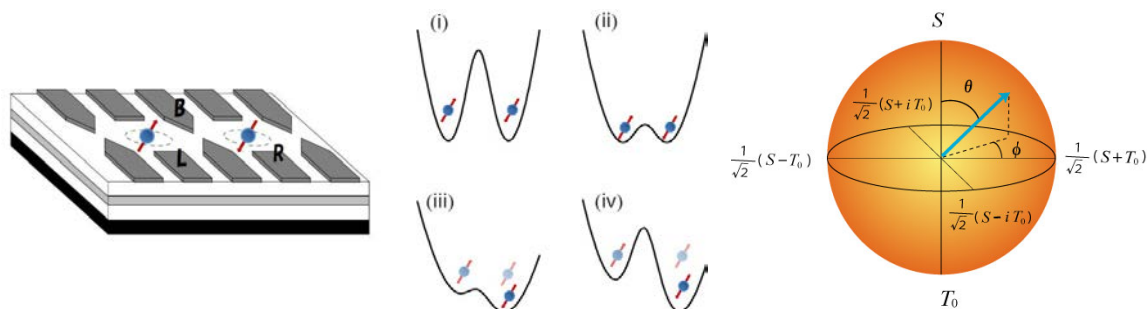
図 3-3. (左) 2 重量子ドットの概念図。青い球が 1 個の電子を、赤い矢印がスピンの向きを、点線は電子が存在し得る範囲を表す。(中) 一連のゲート操作。(i) 測定される 2 電子は初めに左右の量子ドットに 1 つずつ閉じ込めておく。(ii) 中央の障壁を引き下げ、量子ドット間の電子の移動を可能にする。(iii) 電圧をかけることで右の量子ドットにいる電子はスピン-軌道相互作用によるスピン反転を起こしながら確率的に左の量子ドットへ移動する。(iv) 再び障壁を引き上げた後、左右の量子ドットに存在する電子数を測定する。(右) スピン量子ビットのブロッホ球。
