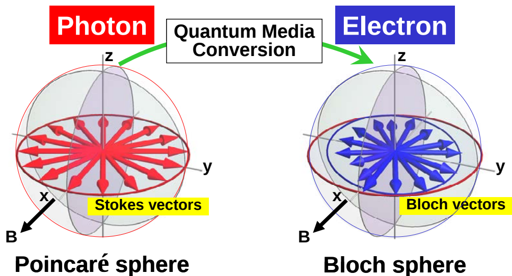
図 1-5. ポアンカレブロッホ球における x-y 面内でのスピン状態転写の実験結果。 g 因子をゼロに設計した井戸厚 6nm の GaAs/AlGaAs 量子井戸を用いてある。実測した g 因子は 0.02 以下である。 z は面直方向を、 x は磁場方向を示す。ブロッホベクトルの長さは最大を 1 に規格化した。
