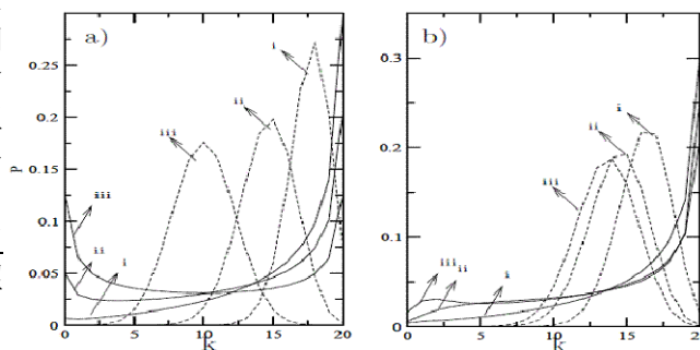
図 4-2. 核スピンの量子メモリ効果を示す計算結果。ゲート制御型量子ドットにおいて 2 個の電子のスピン状態(一重項又は三重項)の観測を、20 回連続して行う場合に、一重項を k -回(三重項は 20-k 回)観測する確率をプロットしたもの。 k=0 は、20 回すべて三重項状態、 k=20 は 20 回すべて一重項状態を観測する場合に対応。実線は核スピンのコヒーレンスが 20 回の観測の間保たれている場合、破線は 1 回の観測ごとに核スピンが熱平衡化されると仮定した場合に対応。i, ii, iii は 2 個の電子を別々のドットに引き離れた状態に保持する時間 t の大小を表わす。核スピンによる有効磁場を表わすパラメーター \sigma を用いて \sigma t = 0.5 (i), 1.5 (ii), \infty (iii) と対応。2 電子間の実効的な交換相互作用を J とし、 J=0 (a)、 J/\sigma=0.5 (b) と選んである。(b) では、一重項状態がエネルギー的に有利なため、一重項状態を観測する確率が三重項状態を観測する確率より高くなっている。
