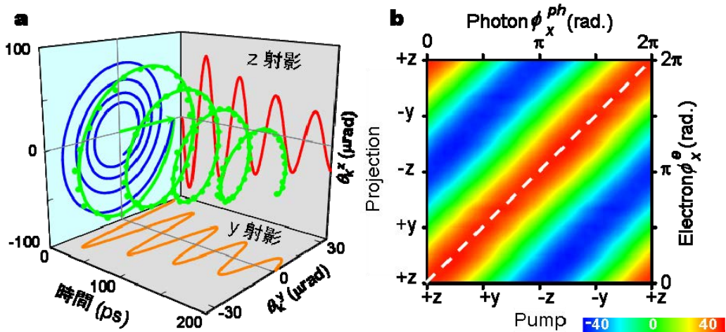
図 1-4. 電子スピン状態トモグラフィ測定の実験結果。(a) 歳差運動する電子スピンの状態ベクトル(ブロッホベクトル)の時間変化。通常のカー回転測定でも測定可能な z 射影に加え、トモグラフィックカー回転測定で初めて可能となった y 射影により、ブロッホベクトルが一意的に確定できる。初期状態は書き込み光の偏光( D^+ )と一致している。(b) トモグラフィックカー回転測定によって明らかになった、書き込み光の偏光コヒーレンスと生成電子のスピンコヒーレンスの対応関係。下軸および上軸はそれぞれ偏光のポアンカレ球上での状態と位相角を、左軸と右軸はそれぞれ電子スピンのブロッホ球上での状態と位相角を示す。破線は両位相が一对一に対応することを示す。
