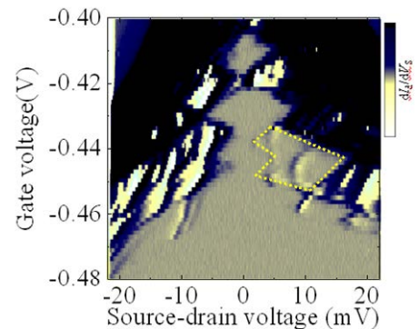
図2-4. InGaAs/InP量子ドットのクーロンダイヤモンド特性。点線で囲まれた領域がスピンプロッケード。
