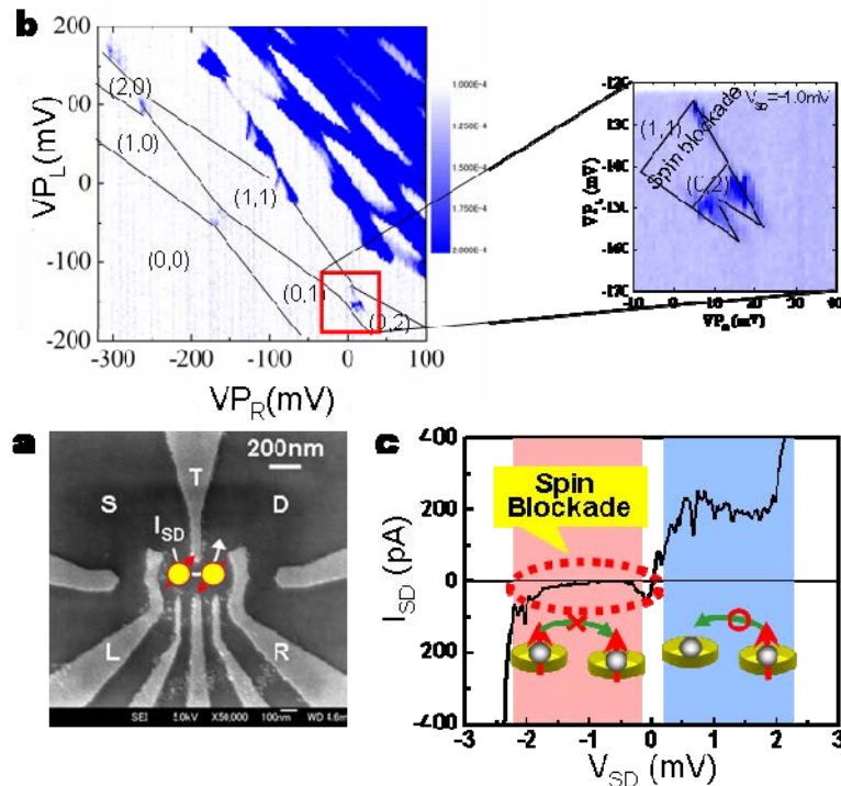
図 1-7. 電子の g 因子をゼロに設計した結合量子ドットにおけるスピンプロッケード現象を利用した電子スピン相関測定。(a) 結合量子ドットのゲート構造 (SEM 写真)。(b) ドット内電子数のゲート電圧による条件設定。拡大領域で電子数が (1, 1) と (0, 2) でほぼ平衡状態となる (c) ドット間貫通電流のソース・ドレイン電圧依存性。ソース・ドレイン電圧に対して電流が非対称となっている。電流の流れない領域がスピンプロッケード現象を示している。この領域では、2 つのドット内の 2 電子相関が三重項状態となっており、パウリ排他律によりスピン緩和するまでの間貫通電流が阻害される。この現象を応用し、光生成した二電子スピン間の量子相関を測定できる。
