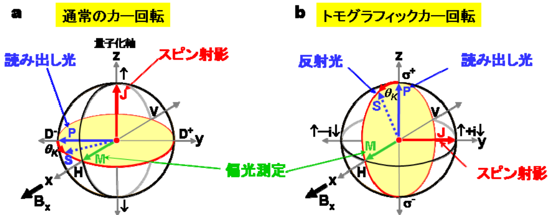
図 1-3. ポアンカレブロッホ球を用いたカー回転測定の説明。(a) 従来のカー回転測定。スピン射影の方向 J は z 方向に限られる。(b) 新たに開発したトモグラフィックカー回転測定。任意の方向 J に射影測定できる。 P はプローブ光の偏光、 S はその散乱（反射）光の偏光、 M は偏光の射影基底を、 J は結果的に測定される電子スピンの射影基底をそれぞれ示す。偏光はあたかも電子スピンによってトルク回転を受けたかのように振舞う。
