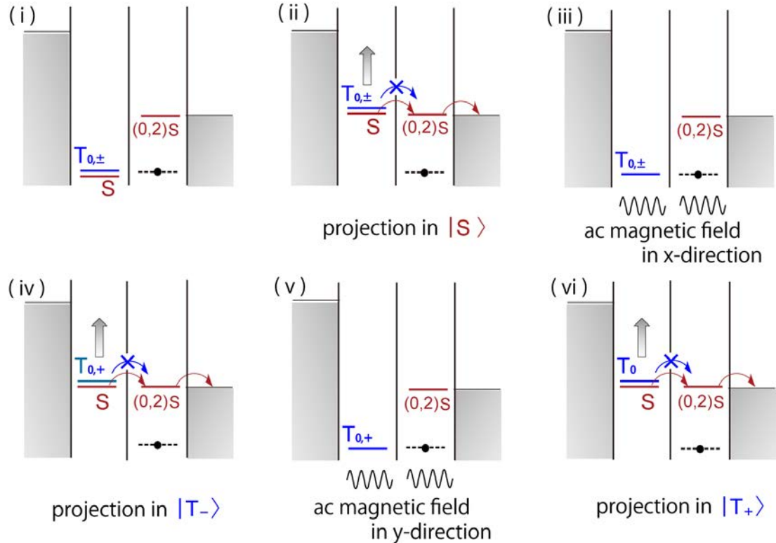
図 3-4. 提案した完全ベル測定の手順を表すエネルギーダイアグラム図。(i) 初期状態。(ii) スピントロニクスを用いてシングレット |S\rangle であるかどうかの測定を行う。(iii) シングレット状態でなければ、x 方向に交流磁場を印加しトリプレット状態の 1 つ |T-\rangle とシングレット |S\rangle とを入れ替える。(iv) スピントロニクスを用いて |S\rangle の測定を行う。この測定で量子ドット内のスピン状態が |S\rangle であると分かると、初期状態が |T-\rangle であったことが分かる。(v, vi) 同様の手順により初期状態が |T+\rangle であったかどうかを測定する。
