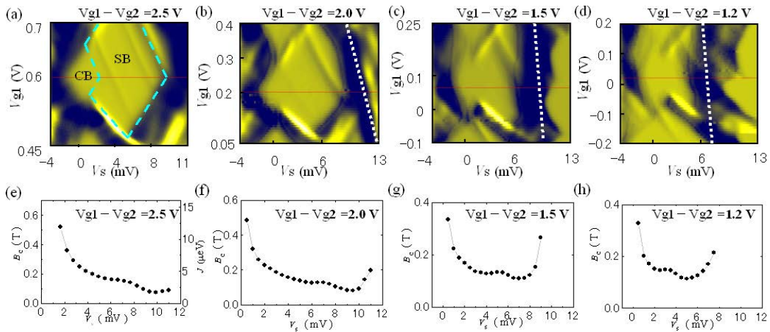
図2-6. 各ゲート電圧におけるスピントロケード近傍の様子 (a-d) と B_c の V_s 依存性 (e-h)
