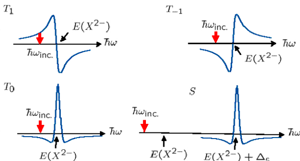
図4-1. 直線偏光のプロブ光に対するFaraday(Kerr)回転角のプロブ光エネルギー( \hbar\omega )依存性。 E(X2^-) は荷電励起子のエネルギー。singlet状態Sに対する共鳴は、 E(X2^-) より軌道状態の励起エネルギー( \Delta e )だけ高エネルギー側に現れる。例えば、プロブ光のエネルギー位置を矢印の位置に選ぶと、2電子のスピン状態(singlet状態S、triplet状態 T_1 , T_0 , T_{-1} )を区別できる。
