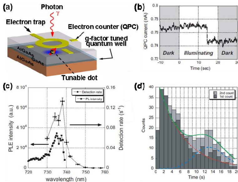
図 1-6. (a) 量子ドットと量子ポイントコンタクト（QPC）からなる量子メディア変換素子。ドット中の電子 g 因子をゼロに制御した量子井戸を持つ。(b) QPC 電流の量子ドットへの光生成電子捕獲による急峻な減少。(c) 光生成電子検出頻度の波長依存（右軸）と同一試料の発光励起スペクトル（左軸）。励起子ピークがほぼ一致する。(d) 一回目（赤線）および二回目（青線）の光子吸収時間の頻度プロット。これらの頻度分布の相違は量子ドット内の二電子相関を反映している。
