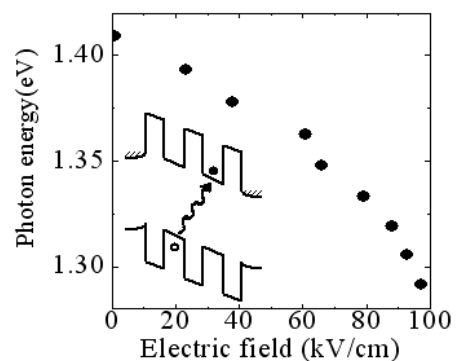
図2-1. 縦型2重ドットにおける間接励起子吸収 (挿入図) と間接励起子吸収端における光子エネルギーの電界依存性。
