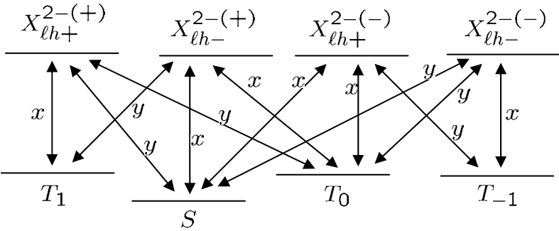
図 4-3. 2 電子のスピンの状態を回転するための光学遷移の選択則。量子ドットが形成される量子井戸面に平行に磁場が印加され (Voigt 配置)、光は井戸面に垂直に入射する (z-方向)。X 2- lh は 3 個の電子と 1 個の軽い正孔からなる荷電励起子状態、(+), (-) は、励起状態にある 3 個目の電子のスピンの向きを表わす。x, y は偏光方向を表わす。
