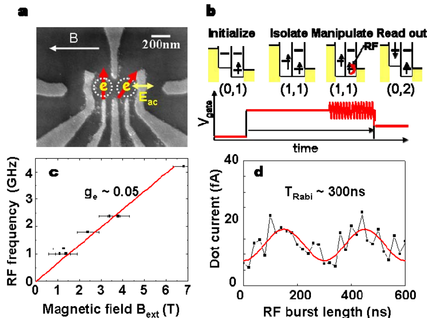
図 1-8. 電子の g 因子を通常より一桁小さく制御した結合二重量子ドットを用いた単一電子スピン操作の実験。(a) 素子構造と磁場方位。右側のゲート電圧を高周波変調し、右側ドットの電子スピンを回転操作する。ドット間を貫通する電流を測定し、二電子相関を評価する。(b) 初期化・操作・読み出しのためのゲート電圧のパルスシーケンス。(c) 単一電子共鳴を示す共鳴周波数の磁場依存性。(d) コヒーレント振動（ラビ振動）を示すドット間貫通電流の高周波パルス幅依存性。
