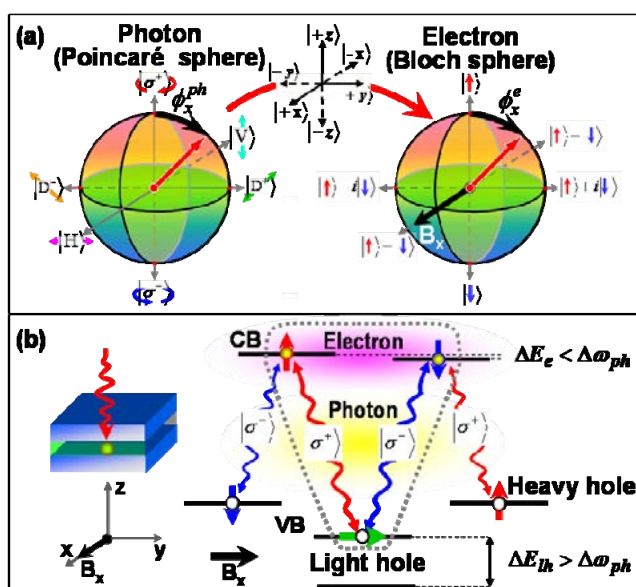
図 1-1. 光子から電子スピンへの量子状態転写の仕組み (a) と転写に必要なバンド構造の条件 (b)。
