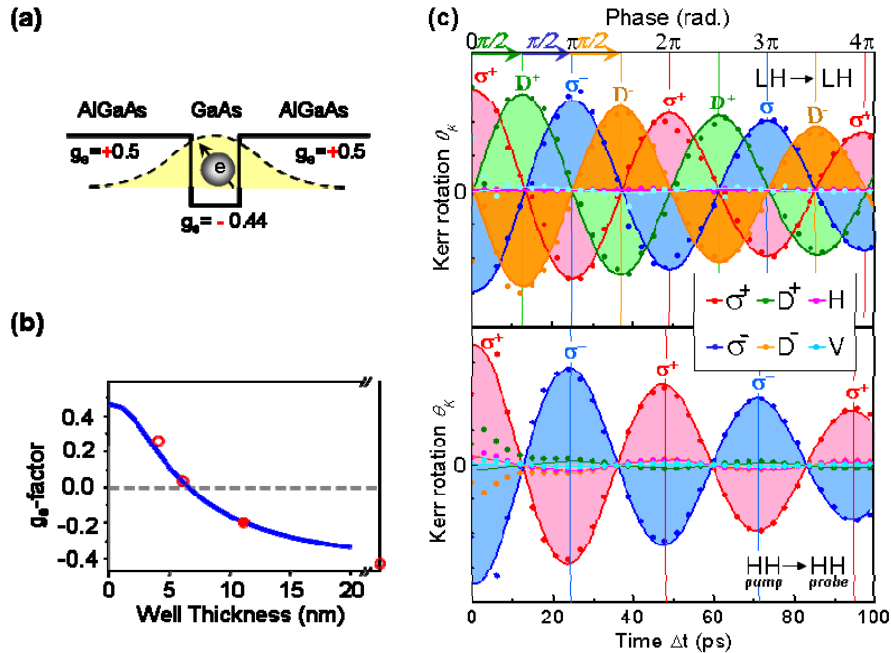
図 1-2. (a) 量子井戸構造 (b) g 因子の井戸厚依存性 (c) 量子状態転写の実証をするための時間分解カー回転の実験結果。上段はポンプ、プローブともに軽い正孔励起子を生成する波長の場合。下段はともに重い正孔励起子を生成する波長の場合。直線偏光 ( D^+ , D^- ) に大きな違いが生じる。
