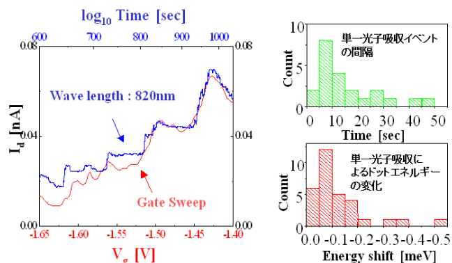
図2-2. 左：ダークにおけるソース・ドレイン電流のゲート依存性 (赤線) および、ゲート電圧固定で820nmの微弱光を照射した際の電流の時間変化 (青線)。離散的な電流の変化が起こる。右：単一光子吸収イベントおよびドットエネルギー変化のヒストグラム。
