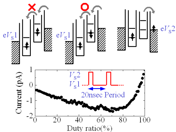
図2-5. スピンブロッケード状態のバイアス電圧 V_{s1} (左上模式図) とそれが解除される電圧 V_{s2} (同右上) との間を20ナノ秒周期でスイッチしたときの過渡電流のデューティ比依存性。中間の領域でスピンが1重項にリセットされることで流れる有限の電流が観測される。
