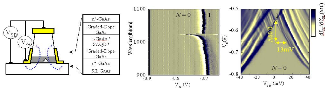
図2-3. 左：InAsドット内包縦型素子模式図と基板の構造。中央電子数1のクーロン振動ピーク位置の照射波長依存性。照射波長・1025nmにおいてクーロンピーク位置が0.09Vシフトする。右：素子のクーロンダイヤモンド特性、ゲート電圧で0.09Vの変化は13meVのドットポテンシャルの変化に相当する。
