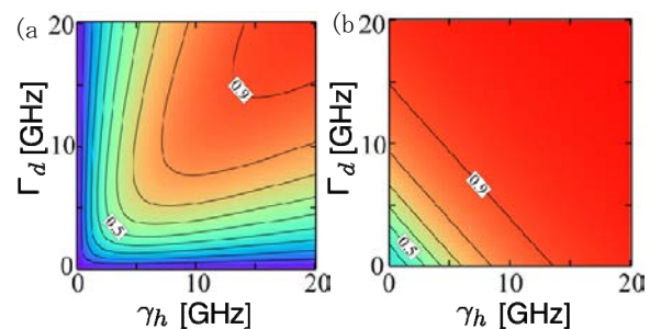
図 3-1. (a) 転写効率及び(b)転写の忠実度のパラメータ依存性。横軸 \gamma_h は正孔の引き抜きレート、縦軸 \Gamma_d は量子ドット-光子間結合強度。対角線上で高い転写効率が得られる(整合条件)。正孔の高速な引き抜きあるいは励起子と光子の強い結合により、忠実度を1に限りなく近づけることができる。
