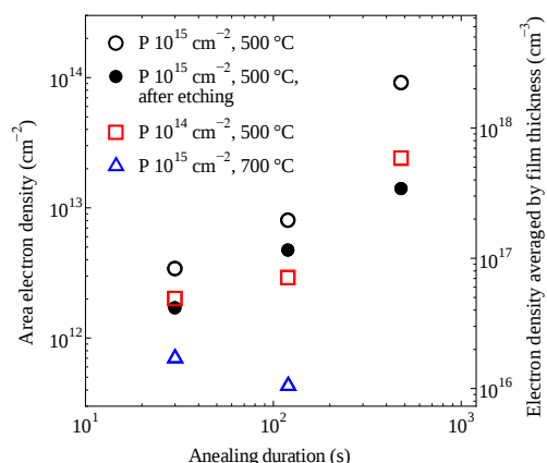
図 31. P ドープ BaSi 2 薄膜における電子密度の活性化アニールによる変化。
