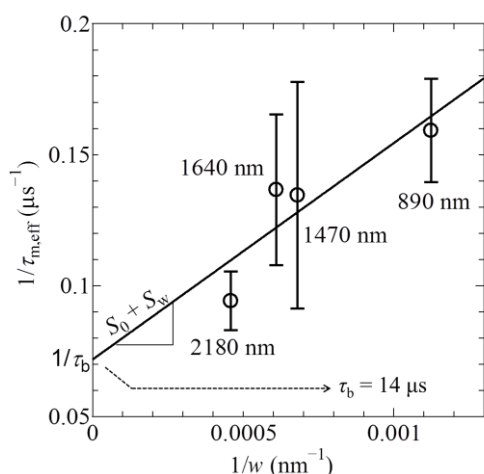
図 39. 膜厚( w )の逆数と実効少数キャリア寿命( \tau_{m,eff} )の逆数の関係を利用したバルク少数キャリア寿命の決定。
