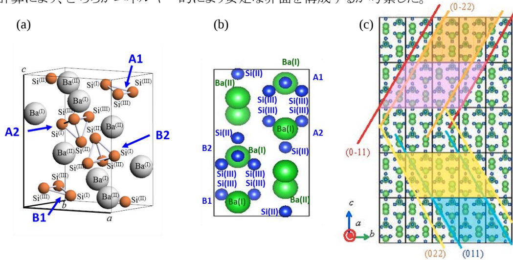
図 11. (a) BaSi 2 ユニットセル。Si(II)Si(III) 2 の 2 等辺三角形底面に対して、Si(I)原子が a 軸正方向にある四面体(B1, B2)と負方向にある四面体(A1, A2)に分類できる。(b) a 軸正方向から見たユニットセル。(c) (011),(0-22)面は Ba(I)原子のみを含み、(0-11),(022)面は、Ba(I)と Si 四面体を含む。
