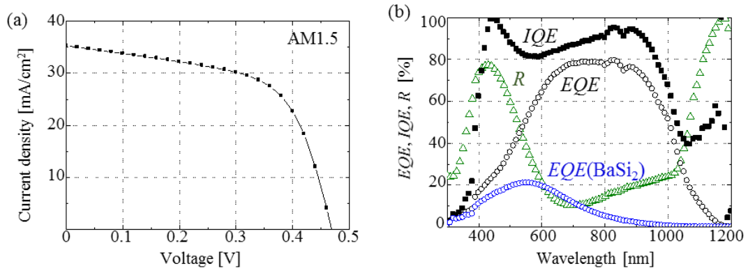
図 28. (a) p-BaSi 2 /n-Si ヘテロ接合ダイオードの AM1.5 照射下での電流密度-電圧特性。 (b) 外部量子効率、内部量子効率、反射率スペクトル。
