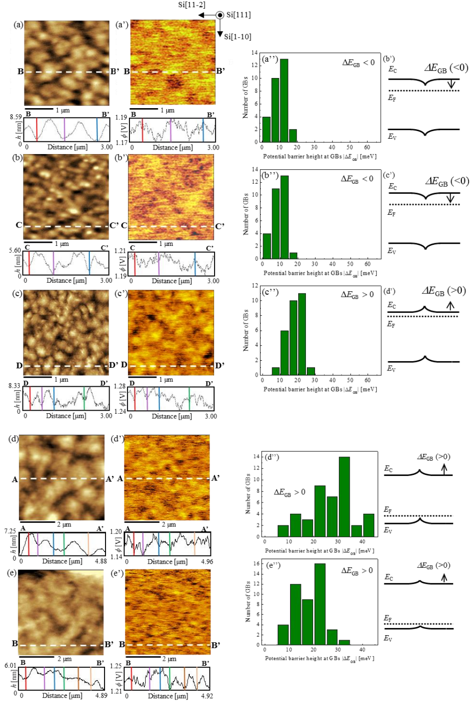
図10. Si(111)面に形成した不純物ドーパドエピタキシャル膜の AFM, KFM 像、障壁高さのヒストグラム。試料のキャリア密度は、(a) n=1.2 \times 10^{17} \text{cm}^{-3} , (b) n=3.2 \times 10^{17} \text{cm}^{-3} , (c) n=1.8 \times 10^{18} \text{cm}^{-3} , (d) p=2.7 \times 10^{18} \text{cm}^{-3} , (e) p=4.0 \times 10^{18} \text{cm}^{-3}
