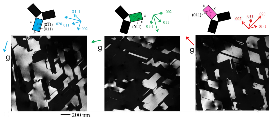
図 6. Si(111)上の a 軸配向 \text{BaSi}_2 エピタキシャル膜について、 g=[004] の二波回折条件で観察した暗視野像。(004)面の回折電子がブラッグ条件を満たす結晶粒が明るく見える。
