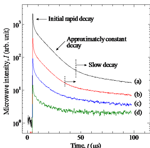
図 36. 異なる励起レーザー強度で評価した 130 nm の BaSi 2 薄膜におけるキャリア減衰挙動。(a) 1.3 \times 10^5 、(b) 1.3 \times 10^4 、(c) 1.1 \times 10^3 、(d) 1.1 \times 10^2 W/cm 2 。
