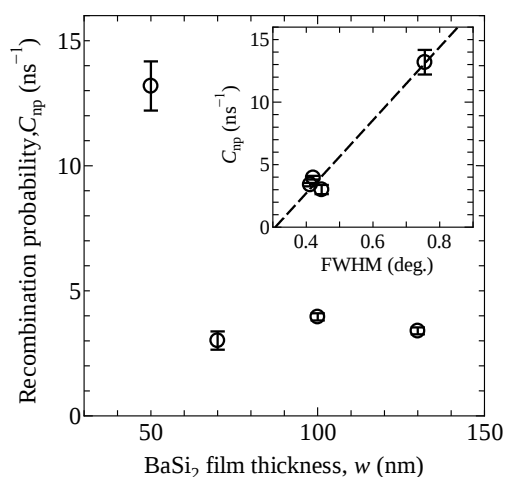
図 37. キャリア捕獲確率( C_{np} )と膜厚( w )、 C_{np} と X 線回折の半値幅(FWHM)の関係。
