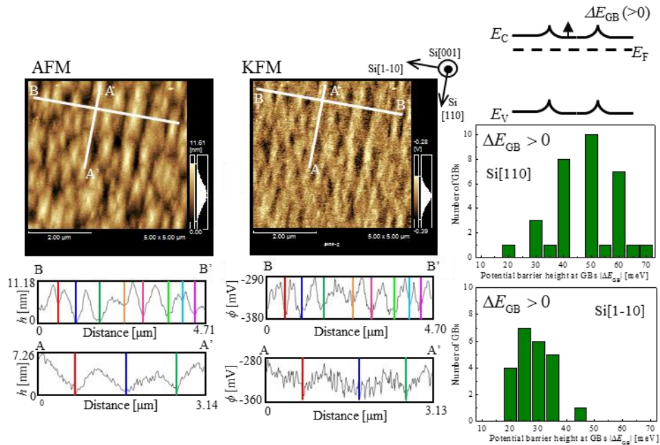
図 9. Si(001)面上アンドープ n-BaSi 2 膜の AFM 像、KFM 像、障壁高さのヒストグラム
