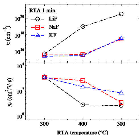
図 34. アルカリ金属フッ化物処理した BaSi 2 薄膜の電子密度と移動度。
