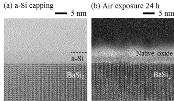
図 18. (a) a-Si/BaSi 2 および(b) ITO/自然酸化膜/BaSi 2 膜の断面 TEM 像。
