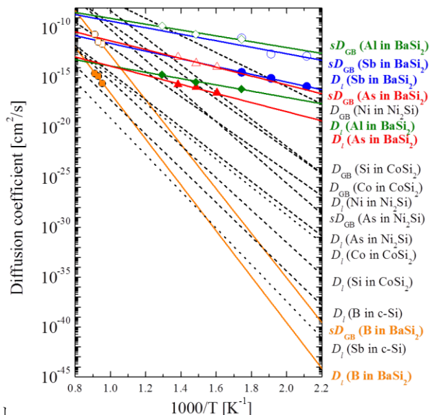
図 23. BaSi 2 エピタキシャル膜中における不純物元素(B, Al, As, Sb)の格子拡散および粒界拡散係数。シリサイド膜および結晶 Si 中の不純物拡散係数も比較のため載せた。
