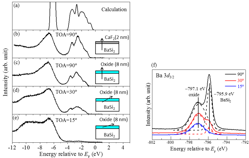
図 17. (a) 計算した HAXPES スペクトル、(b)自然酸化膜の無い \text{CaF}_2 膜でキャップした試料の HAXPES スペクトル、(c)-(e)は自然酸化膜でキャップした HAXPES スペクトルを示す。0eV はフェルミ準位を示す。(b)(c)は試料表面から垂直方向に出てくる光電子を、(d)は試料表面に 30 度の方向、(e)は 15 度の方向に飛び出す光電子を測定した。(f) コアレベル( \text{Ba } 3d_{3/2} )の検出角度依存性。
