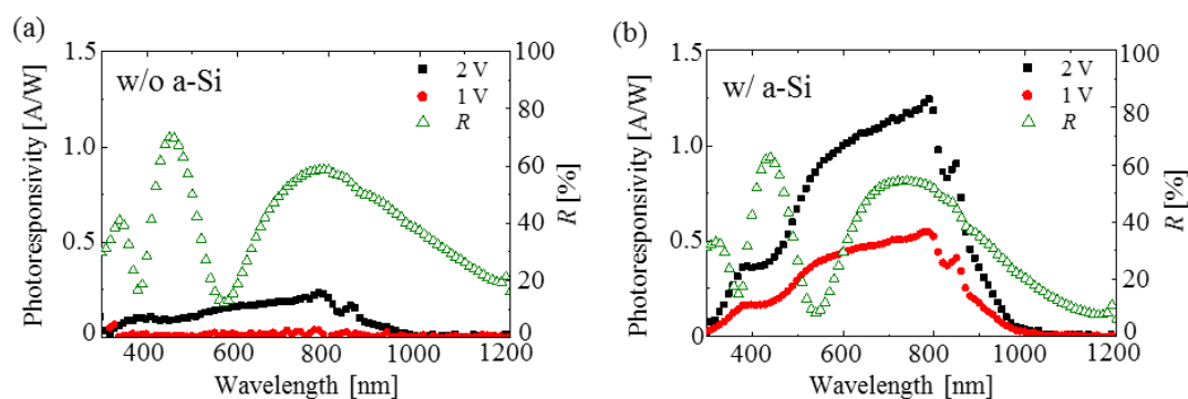
図 20. BaSi 2 膜(500nm)の分光感度特性。(a) は BaSi 2 表面を自然酸化膜で覆った場合、(b) は a-Si 層(5nm)で覆った場合。バイアス電圧を試料表面と裏面に、BaSi 2 膜で生じたホールが自然酸化膜/BaSi 2 界面、または、a-Si/BaSi 2 界面を通過する方向に印加した。
