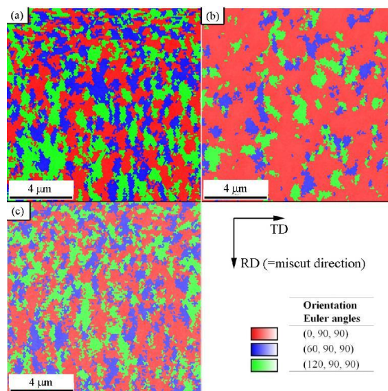
図 35. 微傾斜 Si(111) 基板上 BaSi 2 薄膜の EBSD 方位マップ。傾斜角: (a) 0^\circ 、(b) 2^\circ 、(c) 4^\circ 。
