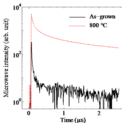
図 38. 800 ^{\circ} C で 30 s のアニールによる余剰キャリア減衰速度の変化。試料膜厚: 3050 nm。
