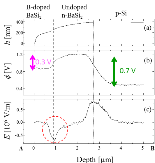
図 24. B ドープ p-BaSi 2 (0.7 μm)/アンドープ n-BaSi 2 膜(1.7 μm)/p-Si(111)構造の断面を用いて測定した、(a)トポ像、(b)ポテンシャル分布、(c) 電場分布。
