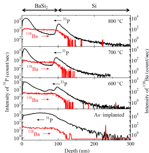
図 30. P 注入 BaSi 2 薄膜における 31 P と 138 Ba の SIMS プロファイルの RTA による変化。
