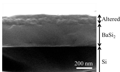
図 32. 高濃度 As 注入( 1 \times 10^{15} \text{ cm}^{-2} )後のアニール(500 °C 1920 s)により変質層が生じた BaSi 2 薄膜の SEM 像。
