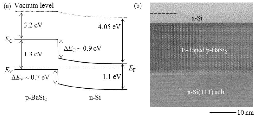
図 27. (a) p-BaSi 2 /n-Si ヘテロ接合ダイオードのバンド構造、 (b) a-Si/p-BaSi 2 (20nm)/n-Si ダイオードの断面 TEM 像。
