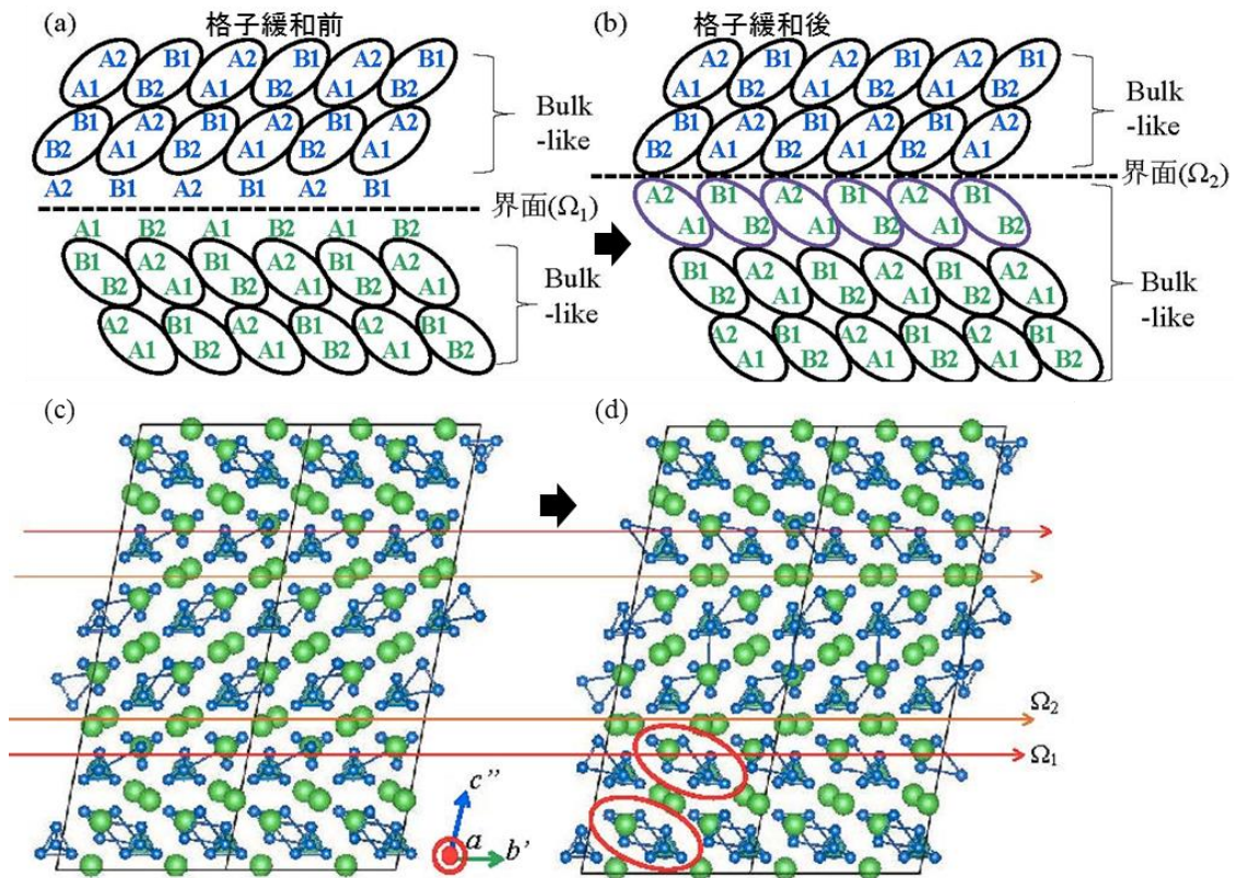
図 13. TypeB 構造の格子緩和前(a)と格子緩和後(b)の粒界付近の Si 四面体ペア。格子緩和後に粒界が \Omega_1 から \Omega_2 に移動したと考えることができる。格子緩和前(c)と格子緩和後(d)の界面付近の原子分布。格子緩和前後における 4.005\text{\AA} 以下のボンド長の分布を表す。格子緩和の前後で、粒界 \Omega_1 の Ba(I)原子の並びが変化している。(d)で粒界が \Omega_1 から \Omega_2 に移動したとすると、Ba(I)で構成される粒界 \Omega_1 を挟んで、120 度回転したバルク結晶が接していると考えられる。粒界 \Omega_2 は Ba(I)で構成される。
