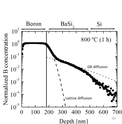
図 22. B/BaSi 2 構造を 800°C で 1 時間アニールした後の B の深さ方向分布。表面側は格子拡散で説明でき、表面から深い領域は粒界拡散で説明できる。
