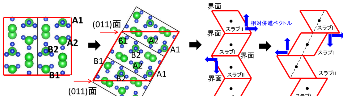
図 12. (011)面を上下表面にもつ表面スラブの形成方法と、これを縦に鏡映関係に組み立てることで粒界を含むスラブモデルを形成する。スラブ I に対して、スラブ II を併進移動した際の粒界エネルギーを計算して、エネルギーが安定する併進操作を見出す。
