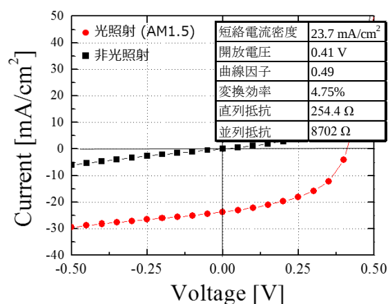
図 25. BaSi 2 -pn 接合ダイオードの電流電圧特性の例。
