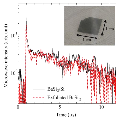
図 41. 800^\circ\text{C} での RTA により歪み緩和した \text{BaSi}_2 薄膜の \mu\text{-PCD} 曲線の、 \text{Si} 基板上で測定した場合と剥離して測定した場合の比較。
