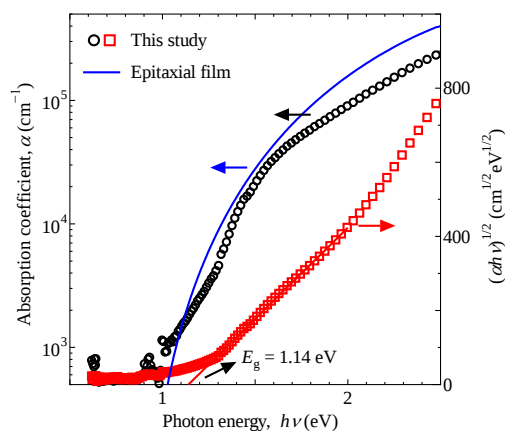
図 43. ガラス基板上 BaSi 2 蒸着膜の光吸収係数と間接遷移吸収端。
