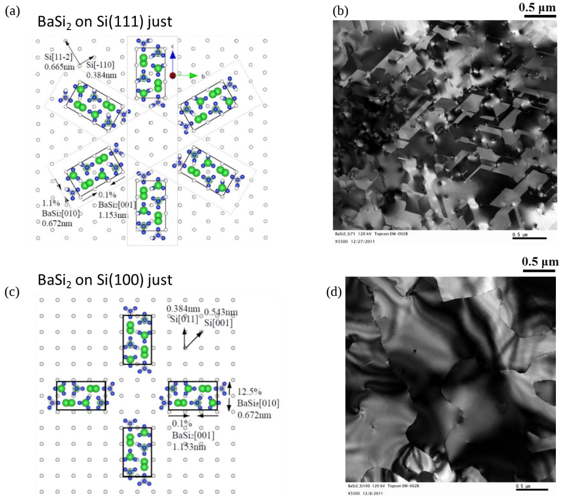
図 5. (a),(b) Si(111)上 BaSi 2 膜のエピタキシャル・モデルと平面 TEM 像。 (c),(d) Si(001)上 BaSi 2 膜のエピタキシャル・モデルと平面 TEM 像。
