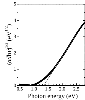
図 3. (\alpha d h \nu)^{1/2} vs E 特性
