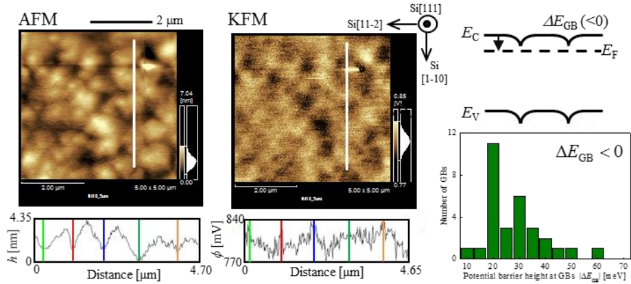
図 8. Si(111)面上アンドープ n-BaSi 2 膜の AFM 像、KFM 像、障壁高さのヒストグラム
