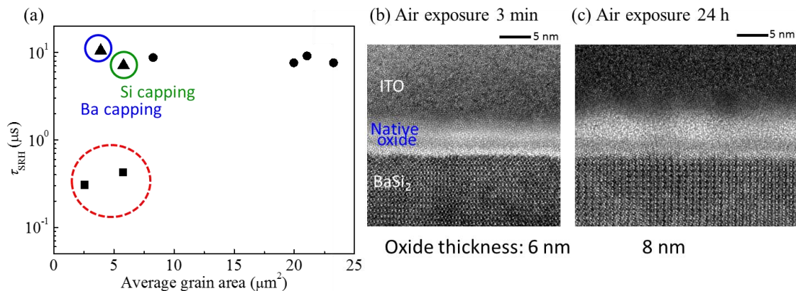
図16. \mu -PCD法で評価した BaSi 2 膜の少数キャリア寿命時間。MBE 成長時の成長条件により、平均粒面積を 3~25 \mu m 2 まで変えた。赤線は、試料表面が鏡面の場合の結果である。(b)(c) ITO/自然酸化膜/BaSi 2 膜の断面 TEM 像。(b)は BaSi 2 成長後の大気暴露時間が 3 分、(c)は 24 時間。
