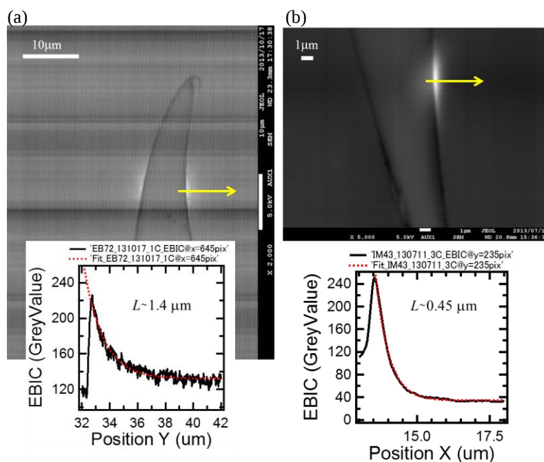
図 7. B ドープ p\text{-BaSi}_2 膜の EBIC 像と矢印に沿う EBIC 強度プロファイル。ホール密度が(a) 10^{17}\text{cm}^{-3} , (b) 10^{18}\text{cm}^{-3} の試料。
