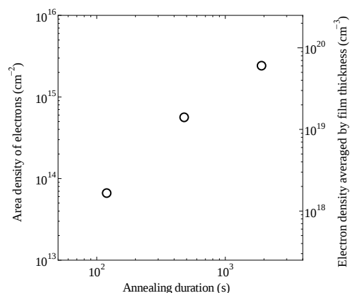
図 33. As ドープ BaSi 2 薄膜における電子密度の活性化アニールによる変化。
