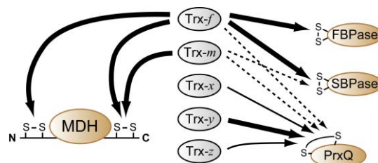
図 2. 葉緑体チオレドキシンアイソフォームの標的特異性 (Yoshida et al. JBC , 2015 より引用)
