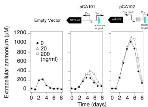
図 7 . GS の発現制御による Anabaena のアンモニア排出 (Higo et al. PCP, 2016 より引用)
