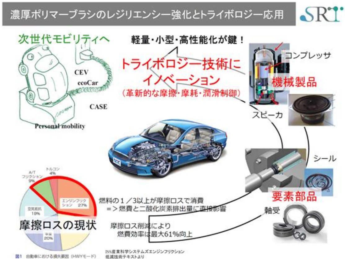
図1 自動車における損失要因 (H/WYモード)
