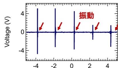
図 3 メンブレン単結晶の振動発電特性。
