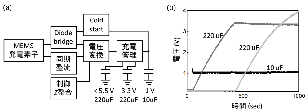
図2: (a)エレクトレット振動発電用の電源回路。(b)試作モジュールの実測結果。3種類の外付けキャパシタが充電されていく様子を示している。
