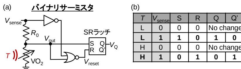
図3: (a)VO 2 を用いたバイナリサーミスタ回路と、(b)温度(T)と印加電圧(V sense )に対する真偽表。V sense = 1 Vを印加したときに、Tが閾値温度より高いか低いかに応じて、SRラッチに値が書き込まれる。
