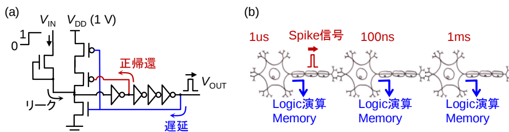
図1: (a)ニューロン回路の回路図。(b)ニューロン回路を用いた「待てるデジタル回路」の模式図。
