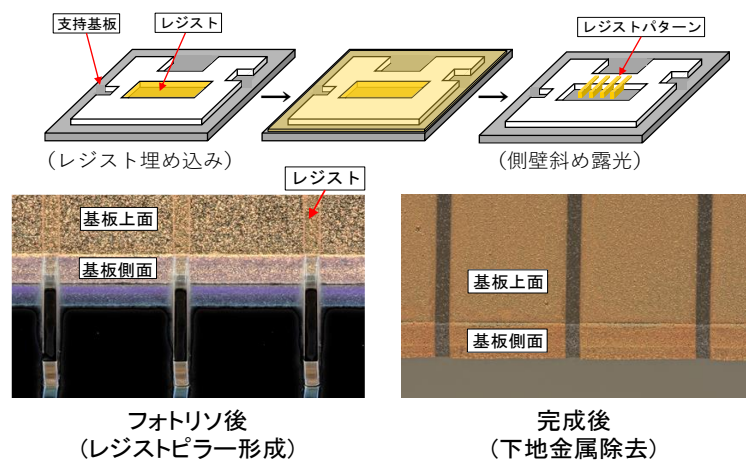
図3 側壁電極パターンの品質改善
