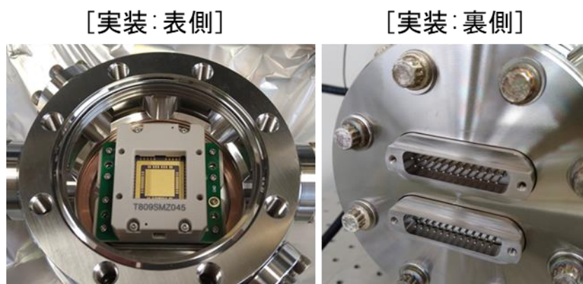
図1 平面型イオントラップパッケージ
