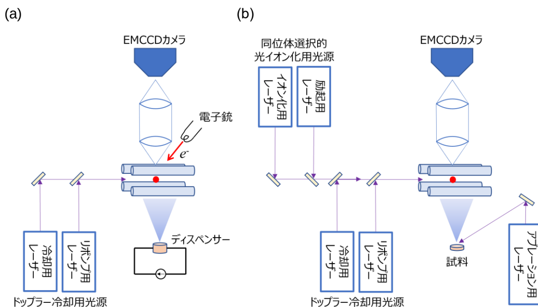
図 1 Ba + 用線形 Paul トラップシステムの概要図。(a)現状のシステム。(b)開発中のシステム。
