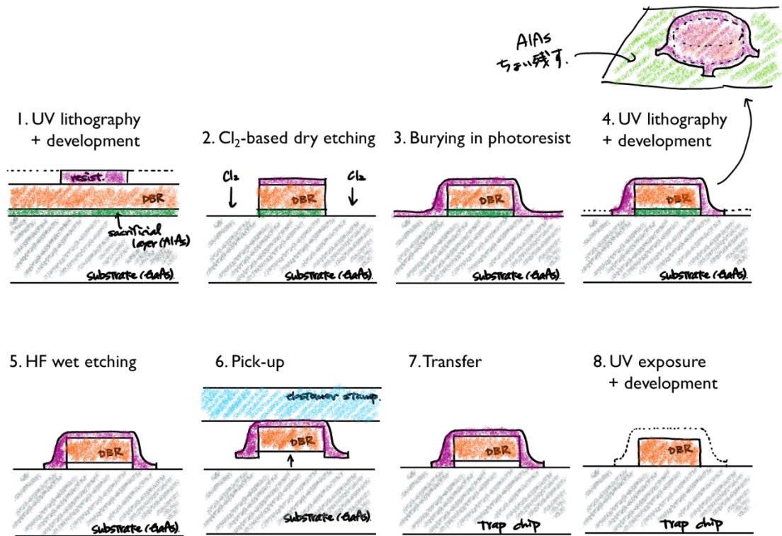
図1 半導体微小ミラーの作製プロセス
