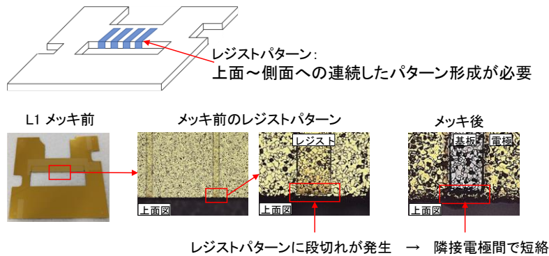
図2 側壁パターンの短絡
