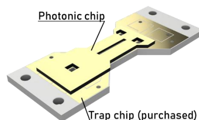
図1 フリップチップ集積による 光回路一体型イオントラップ
