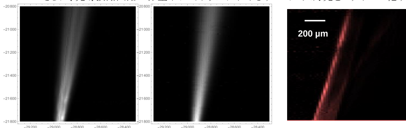
図2 (左)横山研提供の光出射素子の波長 660nm におけるプロファイル (中央)同素子の波長 1092nm におけるプロファイル (右) 作製した光導波路の波長 660nm における出射プロファイル
