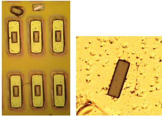
図2 宙吊りになった半導体微小ミラー(左)とトラップチップ上に転写された半導体微小ミラー(右)
