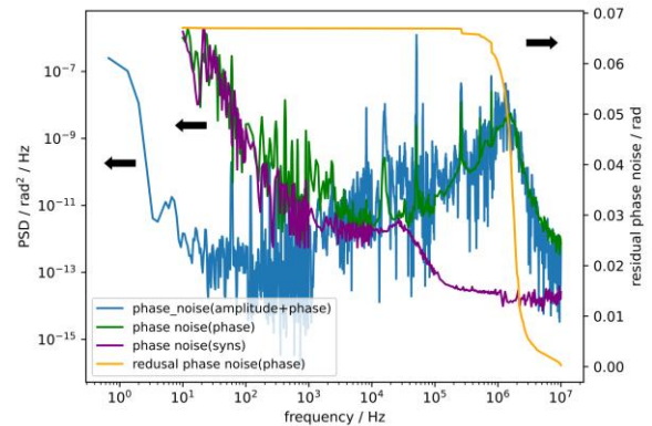
図 2 位相同期中のビート信号の位相雑音 (オレンジ(右の縦軸)が残留位相雑音。他は雑音スペクトル)
