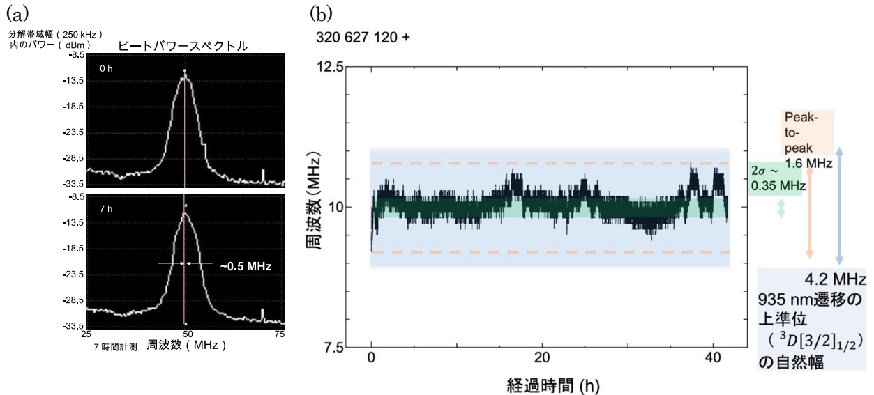
図2 イッテルビウムイオン冷却用光源の周波数安定化実験結果。(a) 935 nm 半導体レーザーを波長計に安定化し、光周波数コムでドリフトを計測した結果。(b) 恒温ブースを動作させたうえで、935 nm 半導体レーザーを光周波数コムに安定化し、安定化 HeNe レーザーで校正した波長計で周波数ドリフトを計測した結果。
