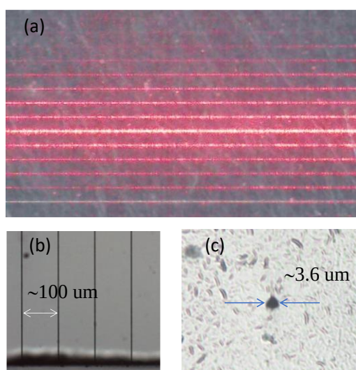
図5 (a) 改質部の光導波の様子。(b) KOH エッチング後の基板内部の高アスペクト比穴構造形成の様子と (c) 穴の断面構造(基板端面の光学顕微鏡像)。
