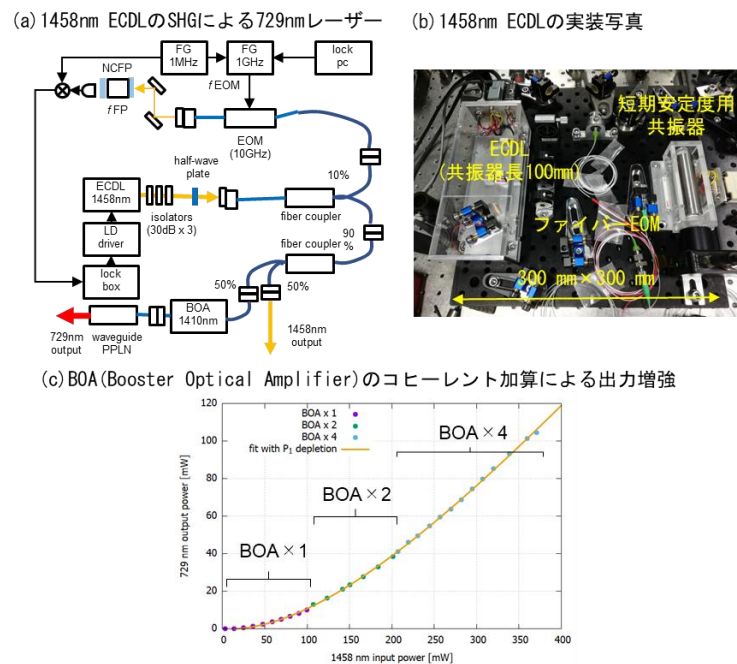
図4 ^{40}\text{Ca}^+ 用 729nm レーザー
