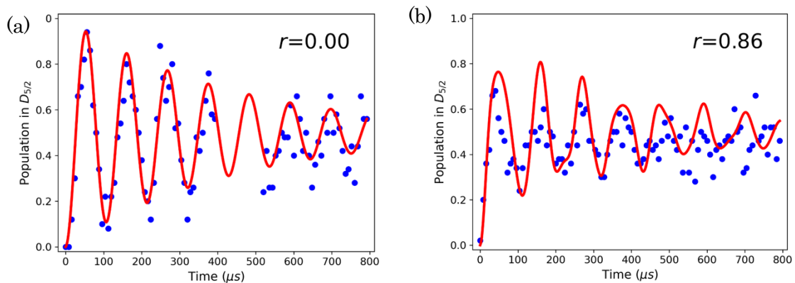
図 1 スクイーズド状態生成実験の結果。(a) スクイージングパラメター r=0 、つまり基底状態生成の場合のブルーサイドバンドラビ振動測定結果。(b) r=0.86 の場合のブルーサイドバンドラビ振動測定結果。
