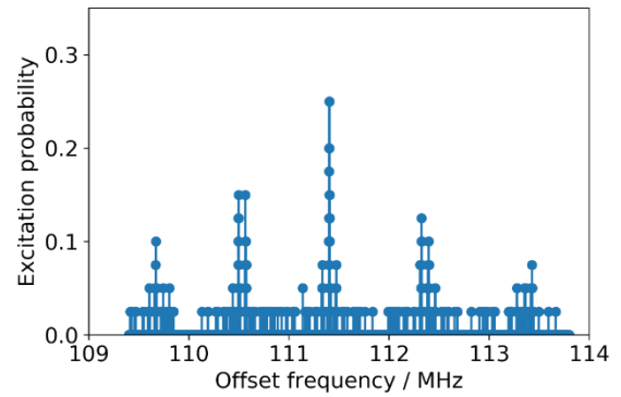
図 1 単一 ^{174}\text{Yb}^+ 2\text{S}_{1/2} - 2\text{D}_{5/2} 遷移のスペクトル
