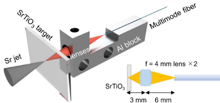
図3 光ファイバーを導波したパルスレーザーによる原子発生の概略図
