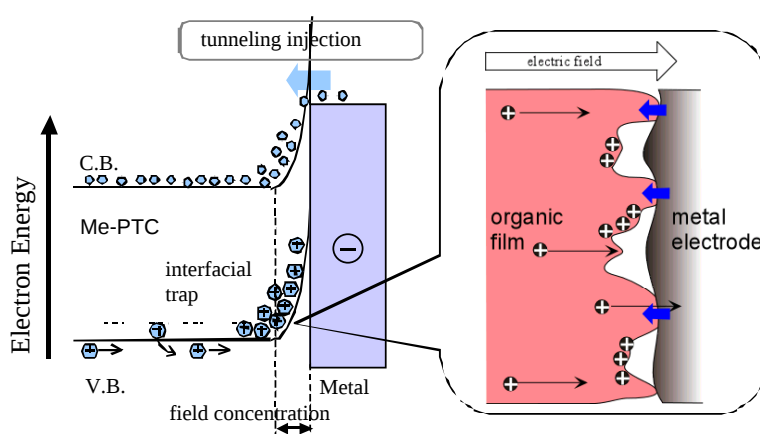
図1 光電流増倍の機構と界面構造トラップ。
