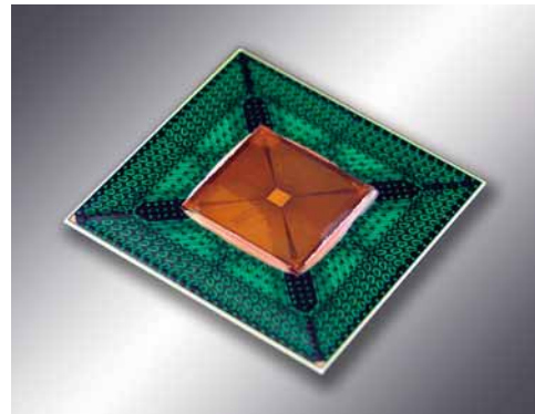
図 10 128×128MOSLM の外観 (FDK 製)
