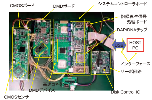
図 73 高速データ転送対応エレクトロニクス(全体構成).
