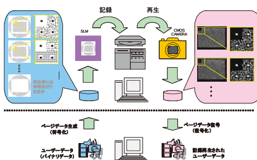
図 61 コリニア方式による動画の記録再生に使用した処理系の構成.
