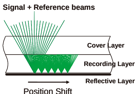
(b) コリニアシフト多重
