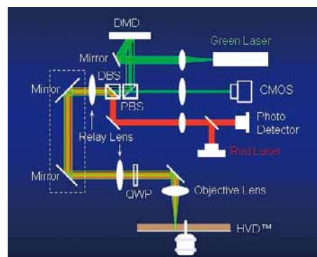
(c) 分離光学系の構成。
