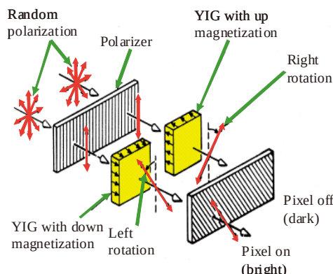
図 16 磁気光学空間光変調器の原理
