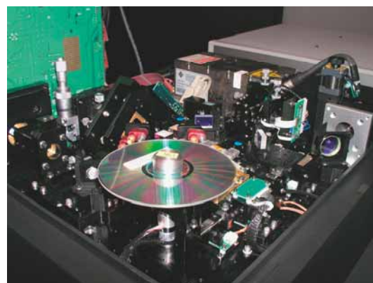
図 13 HVD システムの外観.
