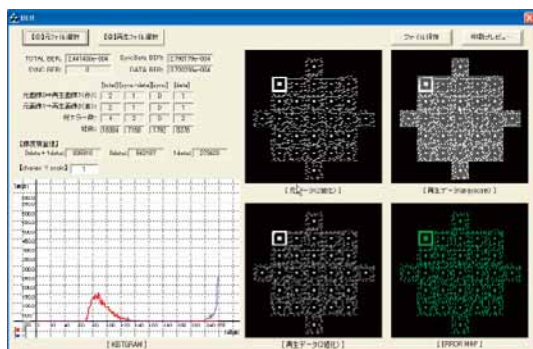
図 32 HUM 方式コリニアホログラムメモリのエラー解析例 (BER, エラーマップ, ヒストグラム表示).
