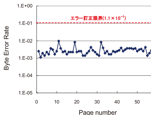
図 34 57 個のページデータの BER 分布 (図 36 の画像データに対応).
