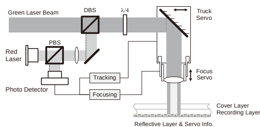
図 53 記録媒体に追従する2軸アクチュエータ部の模式図。
