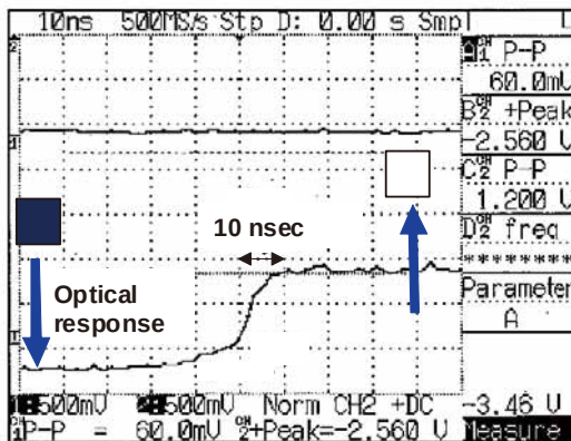
図 9 磁気光学式空間光変調器(MOSLM)のピクセル反転速度
