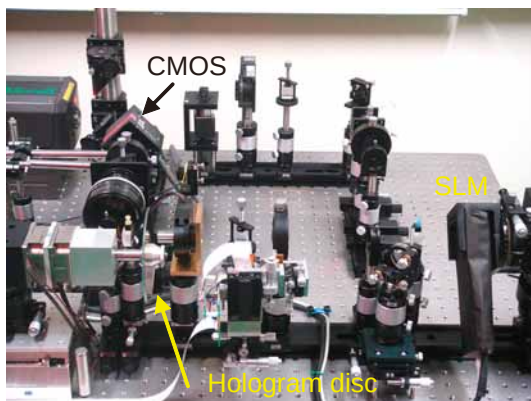
図 30 HUM 方式ホログラムメモリの光学系.
