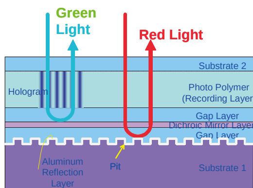
図 54 コリニア方式光ディスクの断面構造。
