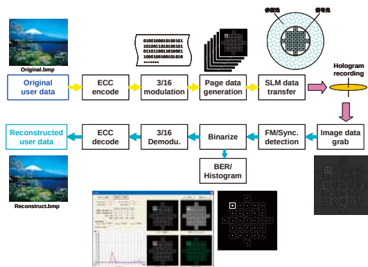
図 31 HUM データ処理のフロー.
