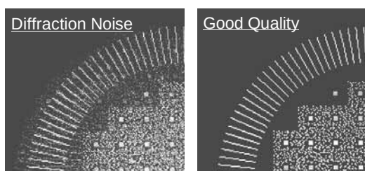
図 55 Dichroic mirror layer の効果。Layer なし(左), Layer あり(右)。
