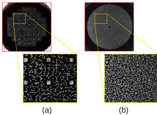
図 73 縮小光学系によるコリニア記録再生結果.(a)は従来の 13.68 \mu\text{m} 角サイズのピクセルを用いた記録再生像, (b)は縮小光学系で 6.84 \mu\text{m} 角サイズのピクセルにして記録再生した再生像.
