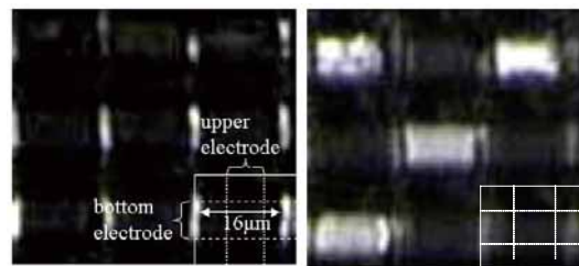
(a) 電圧印加前
