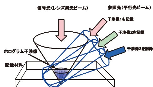
(a) 参照光入射角度を変えて多重(角度多重)
