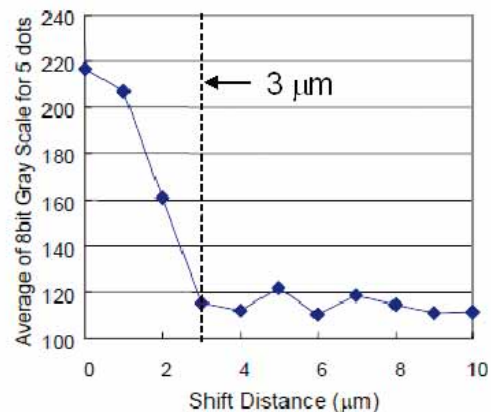
図 24 MOSLM コリニアホログラムシフト選択性.
