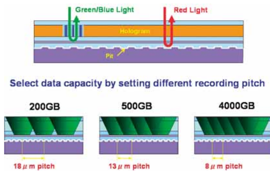
図 76 セレクタブルキャパシティーフォーマット概念図.
