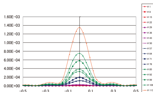
図 37 フッ素系ナノゲルフォトポリマ記録材料の平面波ホログラム測定結果。縦軸は回折効率、横軸はブラッグ角ディチューニング(°)、ディチューニングが0であることは、収縮率が0であることを示す。
