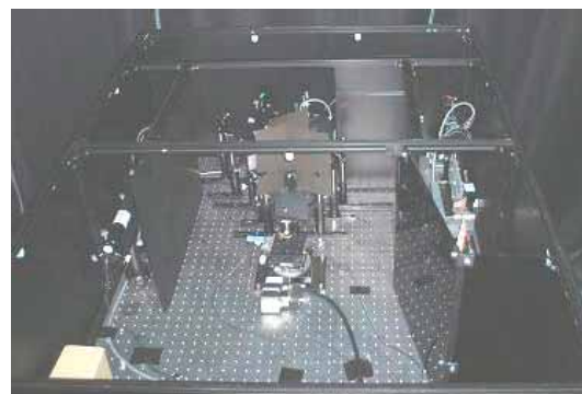
図 38 平面波を用いたホログラム材料評価器(平面波テスター:ハードウェアグループ開発)。
