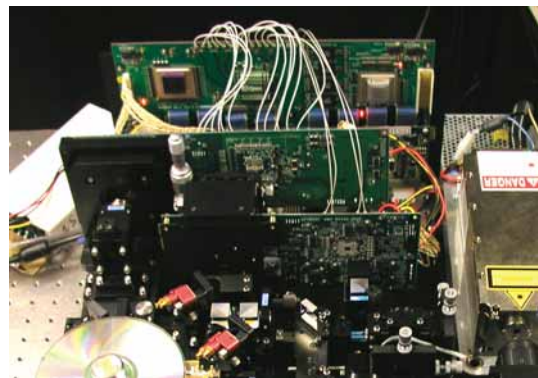
図 74 ES1 に組み込んだ高速データ転送エレクトロニクス.
