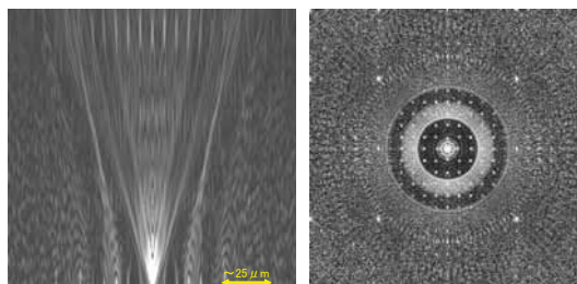
図 51 コリニア方式で記録媒体中に形成される干渉縞の計算結果の一例。記録媒体厚み方向の強度分布(左)とレンズ焦点面における光軸中心の面内強度分布(右)。
