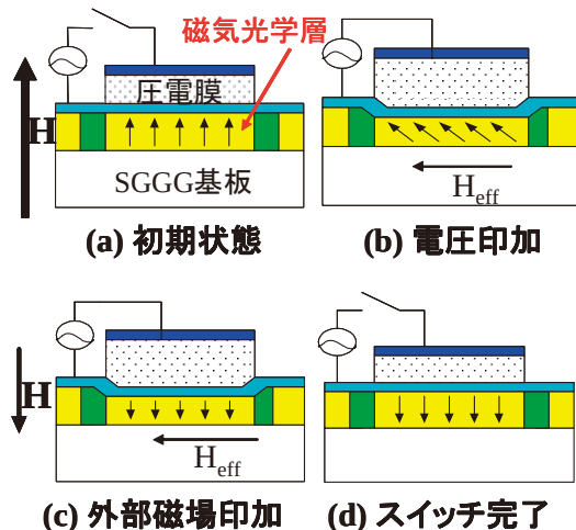
図 25 電圧駆動 MOSLM の原理.
