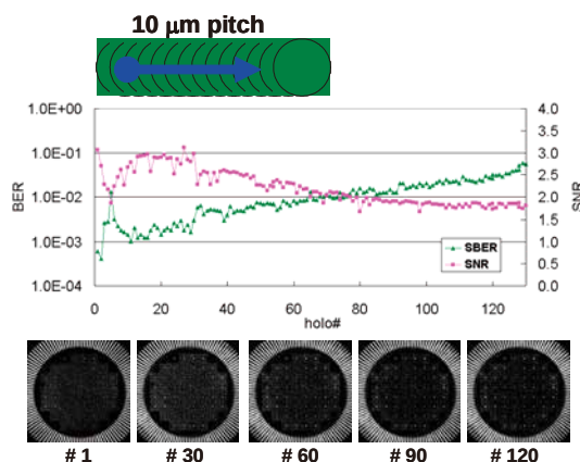
図 44 130 個のホログラムのコリニアシフト多重(シフト間隔は 10 \mu\text{m} ).
