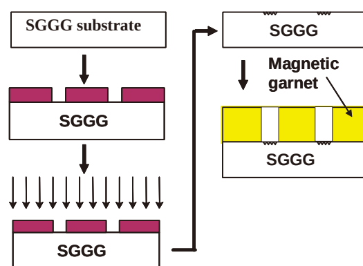
図 18 選択的 LPE 成長によるピクセル形成。
