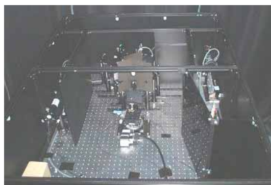
図 12 ホログラム材料テスト.
