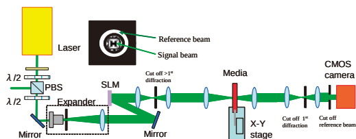
(a) 透過型コリニアホログラフィー光学系
