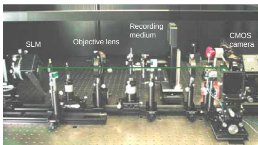
(b) 実際の光学系
