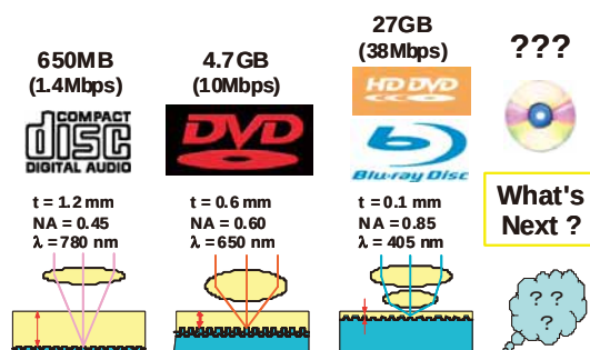
図 1 光ディスク技術の変遷
