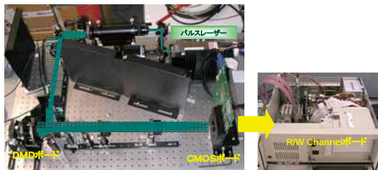
図 67 ページデータの高速伝送と信号処理。
