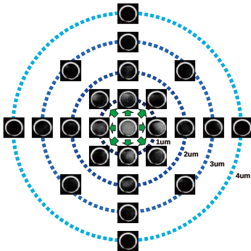
図 8 コリニアシフト多重とクロストーク (Aprilis 製フォトポリマ材料を利用)。
