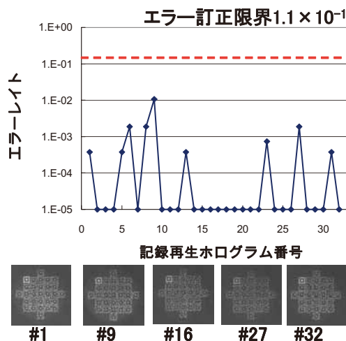
図 47 HUM 方式記録再生結果.
