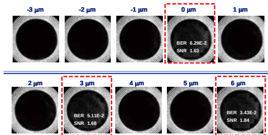
図 43 コリニアシフト多重再生結果. シフト量は 3 \mu\text{m} .
