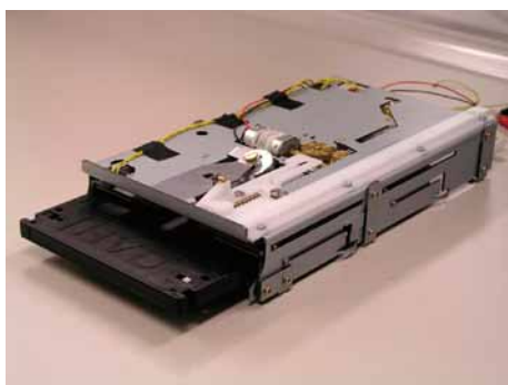
(a) HVD 遮光性カートリッジとローディングメカニズム外観写真.
