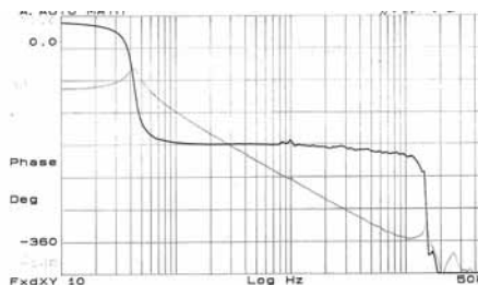
(a) フォーカスサーボ.
