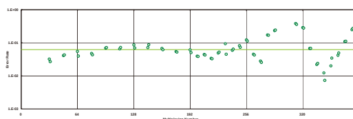
(c) シフトピッチで計算したレイヤー多重数に対するシンボルエラーレート。
