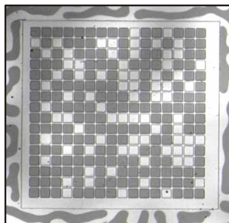
図 17 MOSLM のピクセルイメージ(偏光顕微鏡像)。
