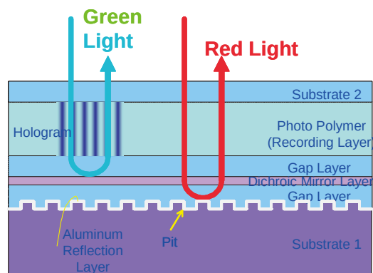
図 14 HVD ホログラムディスクの構造.
