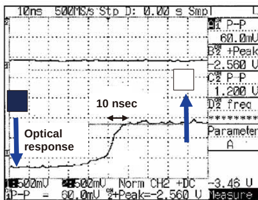
図 21 電流駆動 MOSLM のピクセルスイッチング速度.
