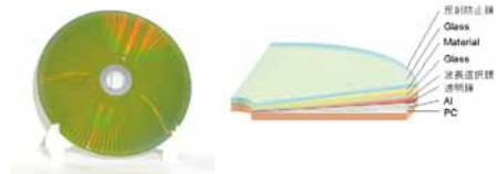
図 46 HUM 及び HVD ホログラム光ディスク.
