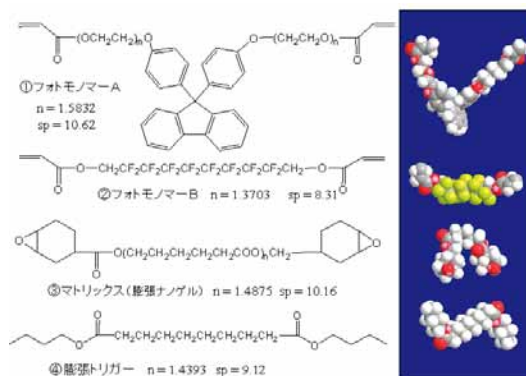
図 35 フッ素系ナノゲルフォトポリマの構成成分の屈折率 n とソルビリティパラメータ sp 値。
