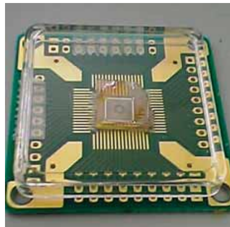
図 28 16 \times 16 電圧駆動 MOSLM プロトタイプ素子.
