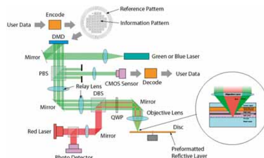
図 52 コリニア方式における二波長光学系の基本構成と動作概要の模式図。
