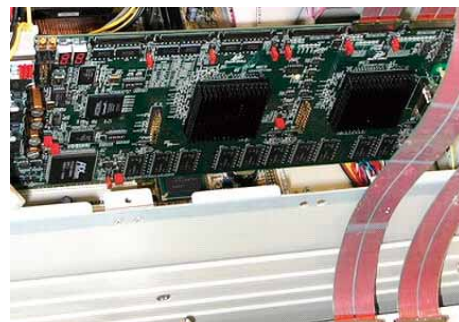
図 66 Enc/Dec 用ハード.
