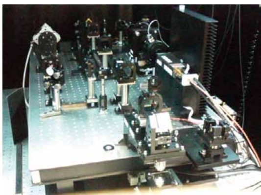
図 40 パルスレーザ光源を用いたコリニアホログラム評価系(反射型).
