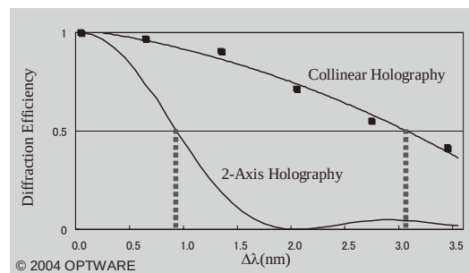
図 57 波長マージン(2光束法との比較)。
