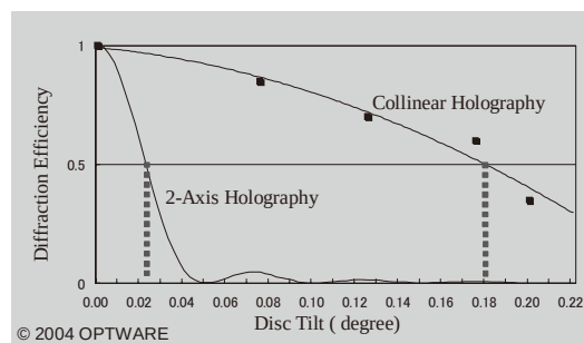
図 56 チルトマージン(2光束法との比較)。
