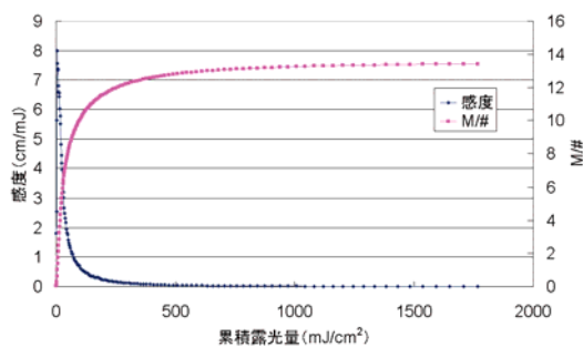
図 39 感度 と M/# の累積露光量依存性.
