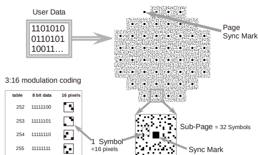
図 50 3-16 変調コーディングと二次元データページフォーマット
