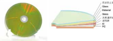
図 15 HUM, HVD ホログラムディスク
