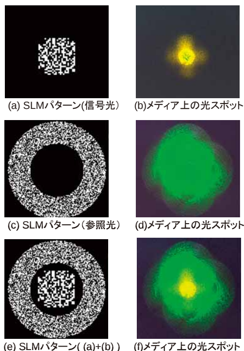
図 6 SLM パターンとメディア上の光スポット
