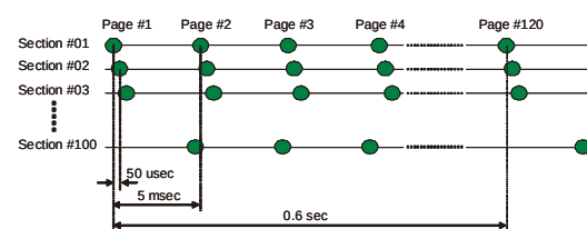
図 62 動画記録再生時の光スポット位置制御.
