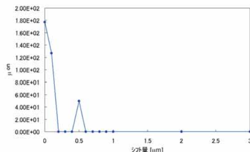
図 42 白ピクセル平均輝度 vs. シフト量.
