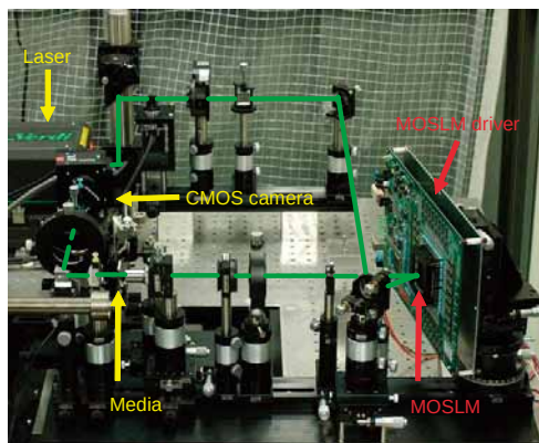
図 22 MOSLM コリニアホログラムテスト光学系(後述の HUM 方式).
