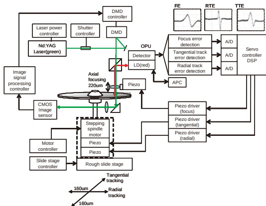
図 29 HUM 方式ホログラムメモリの全体構成ブロック図.
