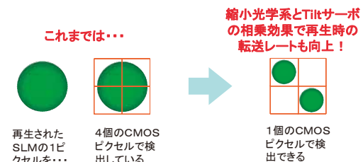
図 75 1 TB/disc, 1 Gbps 達成のアプローチ. 1:1 ピクセルマッチングとディスク面ブレの影響を補正するチルトサーボの融合.
